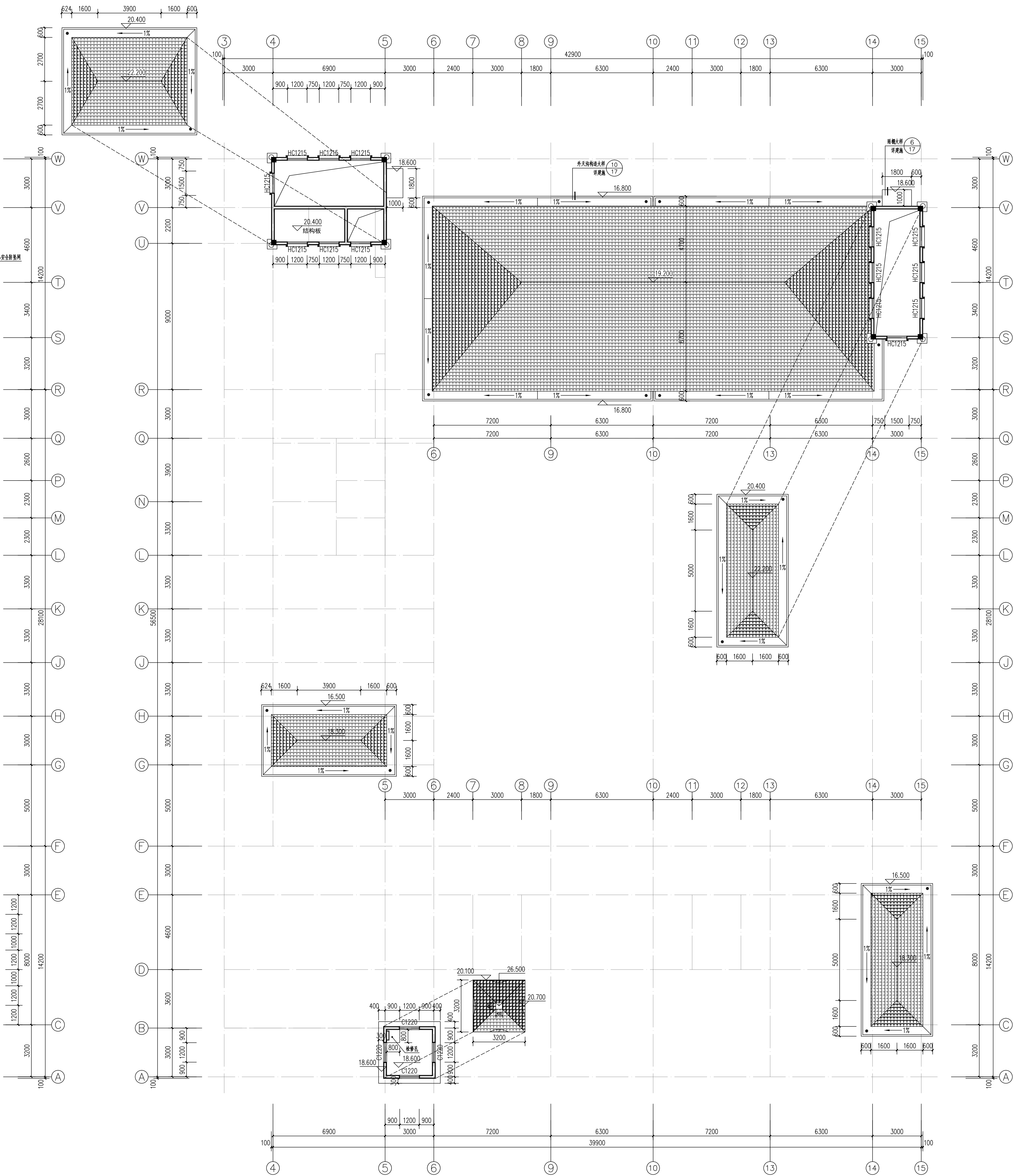
屋面层平面图 1:100
