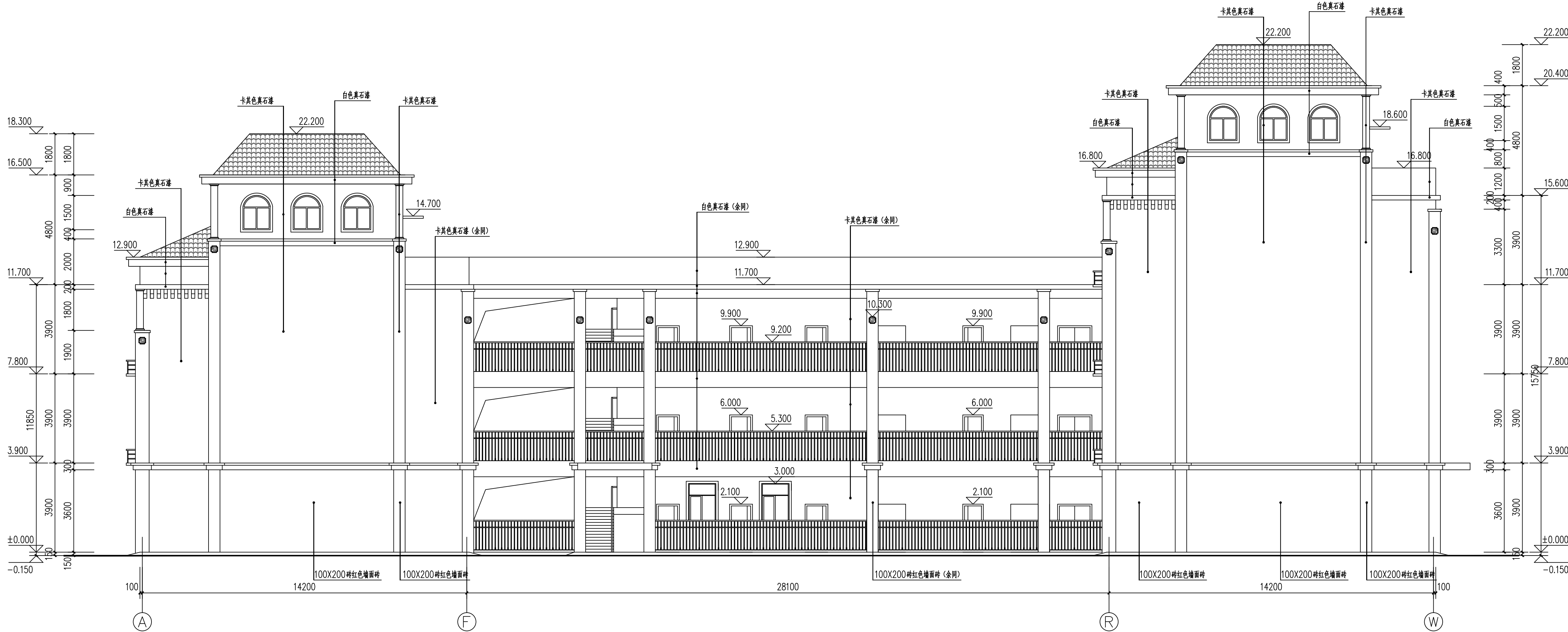
Ⓐ ~ Ⓦ 轴立面图 1:100
