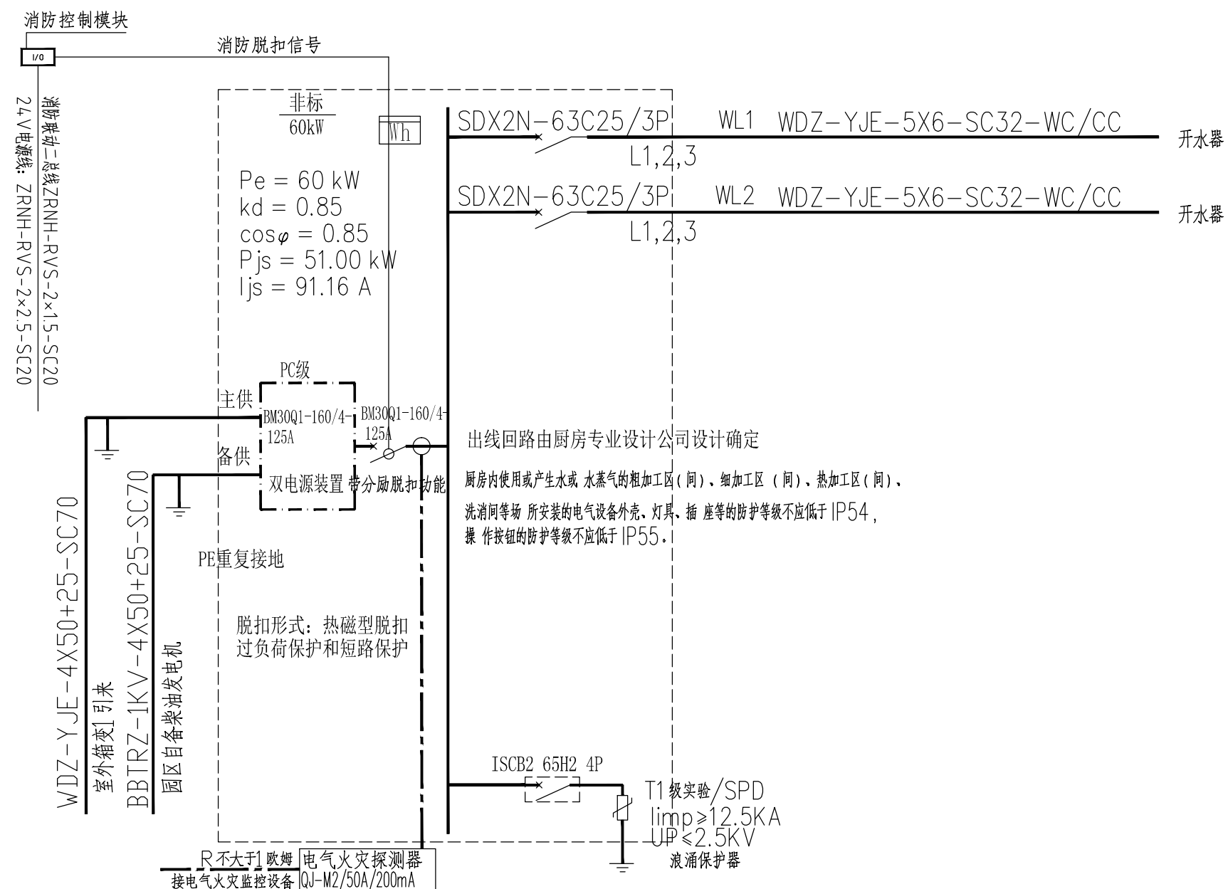
APcf 系统图
