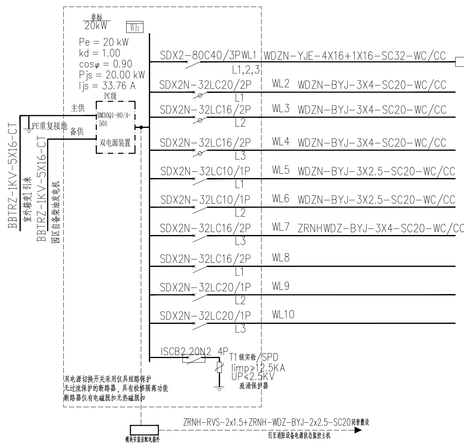
ATxk消防控制室配电系统
