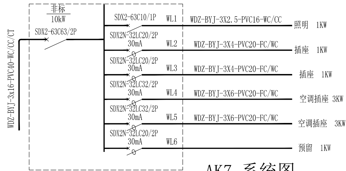
AK7 系统图
