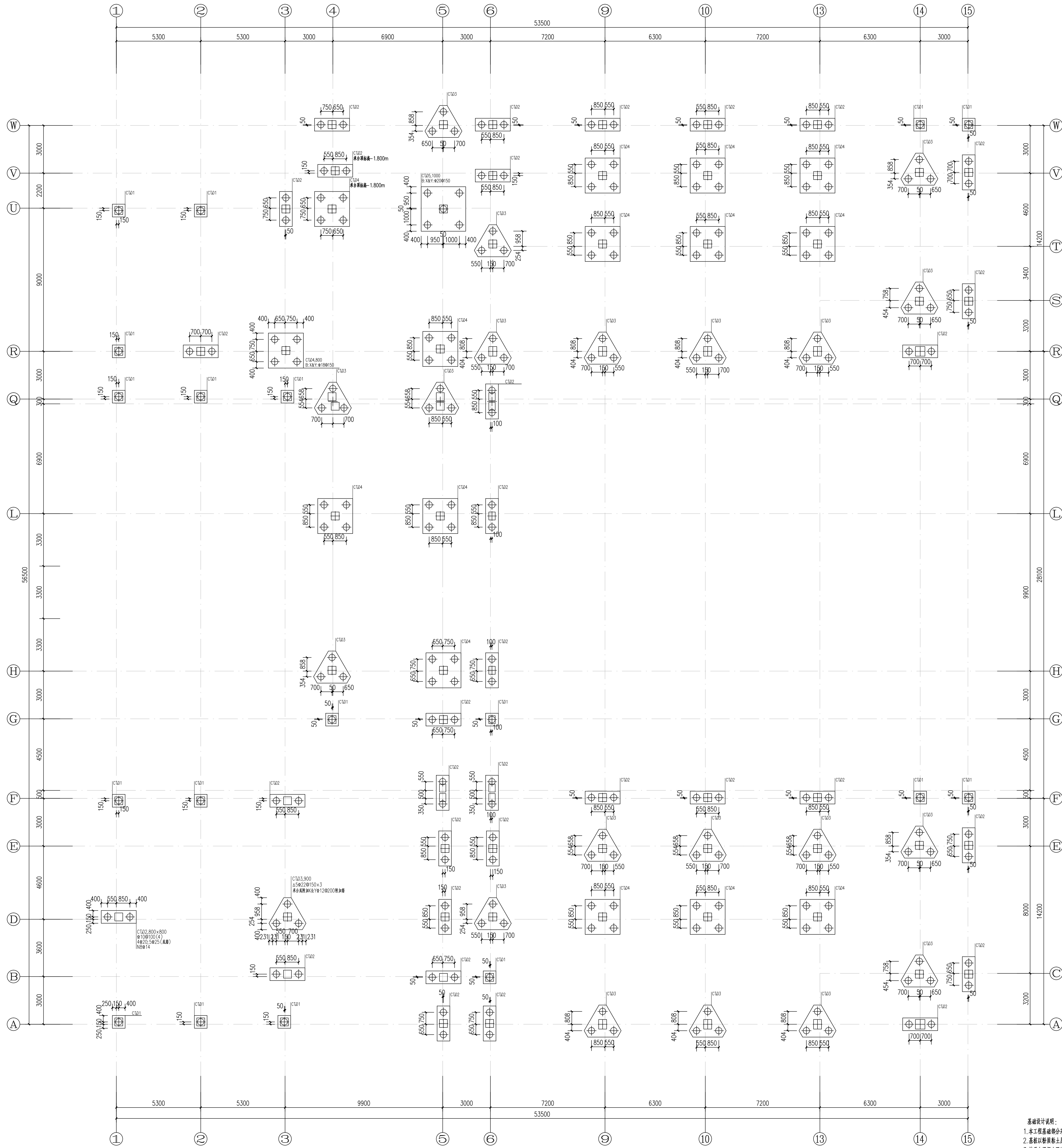
基础平面布置图
