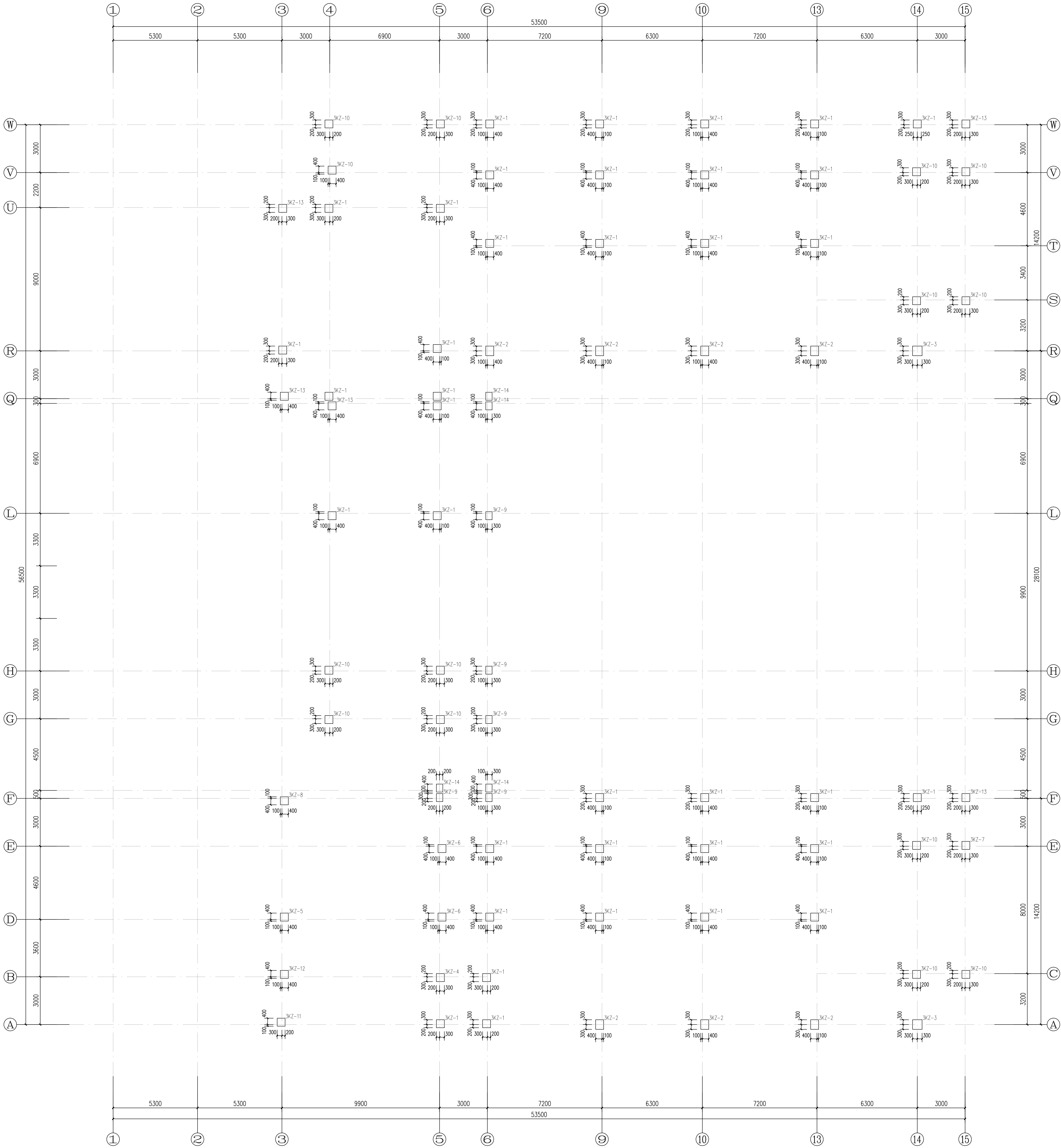
二层柱结构平面图 1. 参照图集 16G101-3
