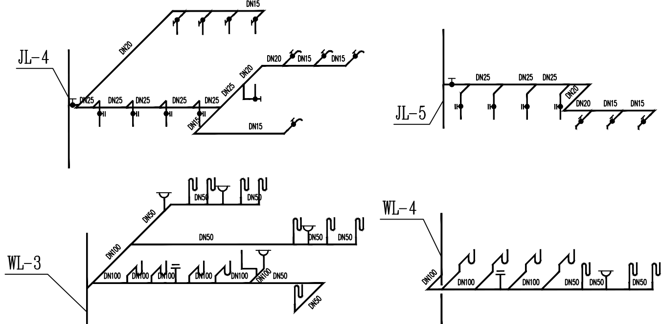
公共卫生间给排水详图
