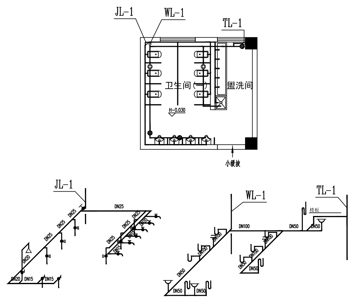
寝室卫生间给排水详图
