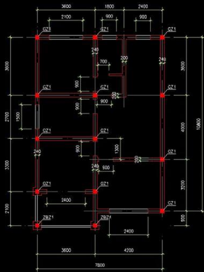
二层墙体布置图
