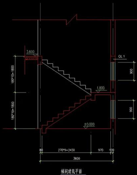
楼梯建筑大样图
