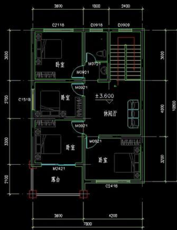
二层建筑平面图
