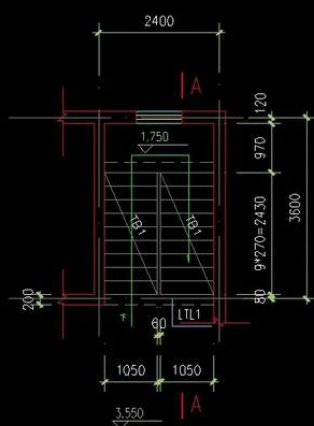
梯间结构平面
