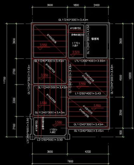
二层结构布置图
