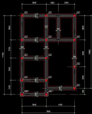
基础结构布置图
