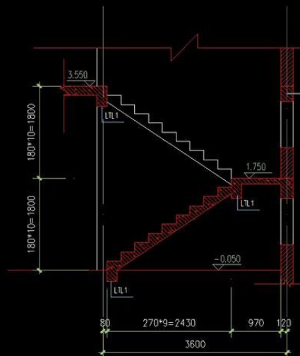
梯间结构剖面
