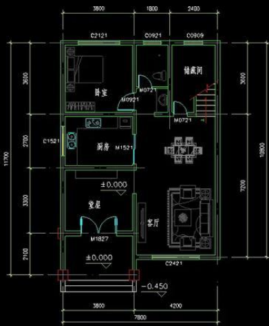
一层建筑平面图
