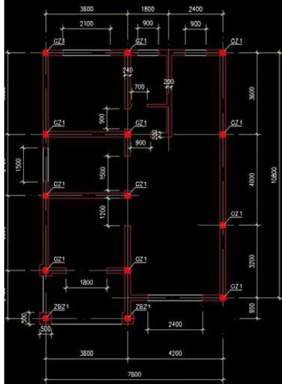
首层墙体布置图
