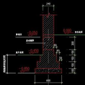
基础大样图
