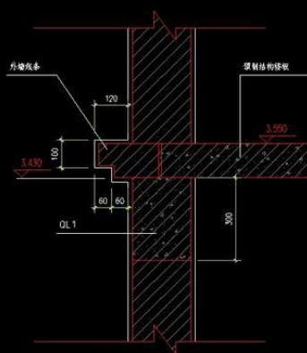
外墙线条大样图
