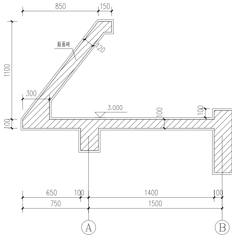
二层构件详图 1:20
