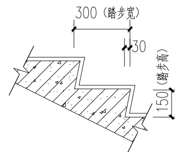
楼梯详图 1:20
