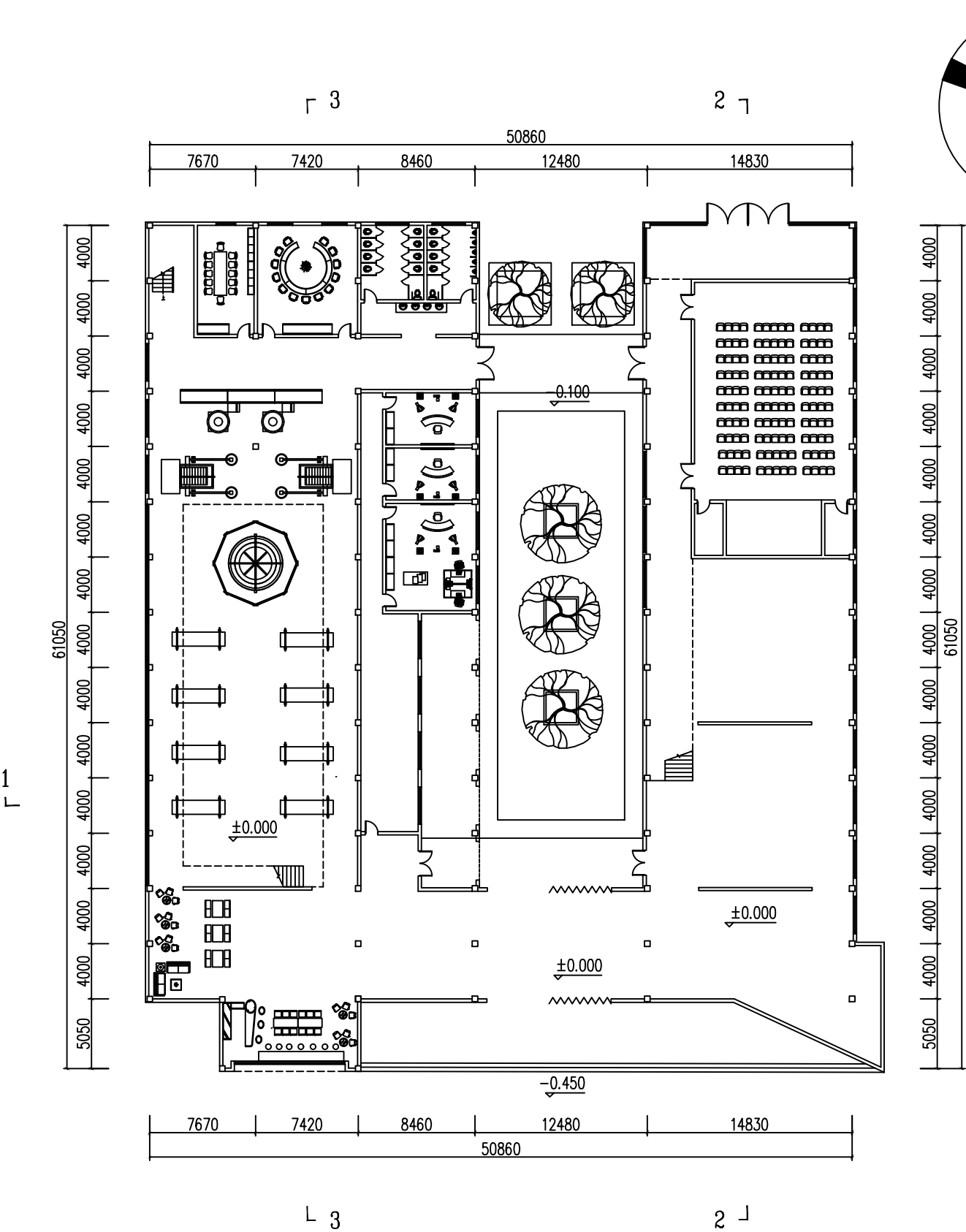
一层平面
