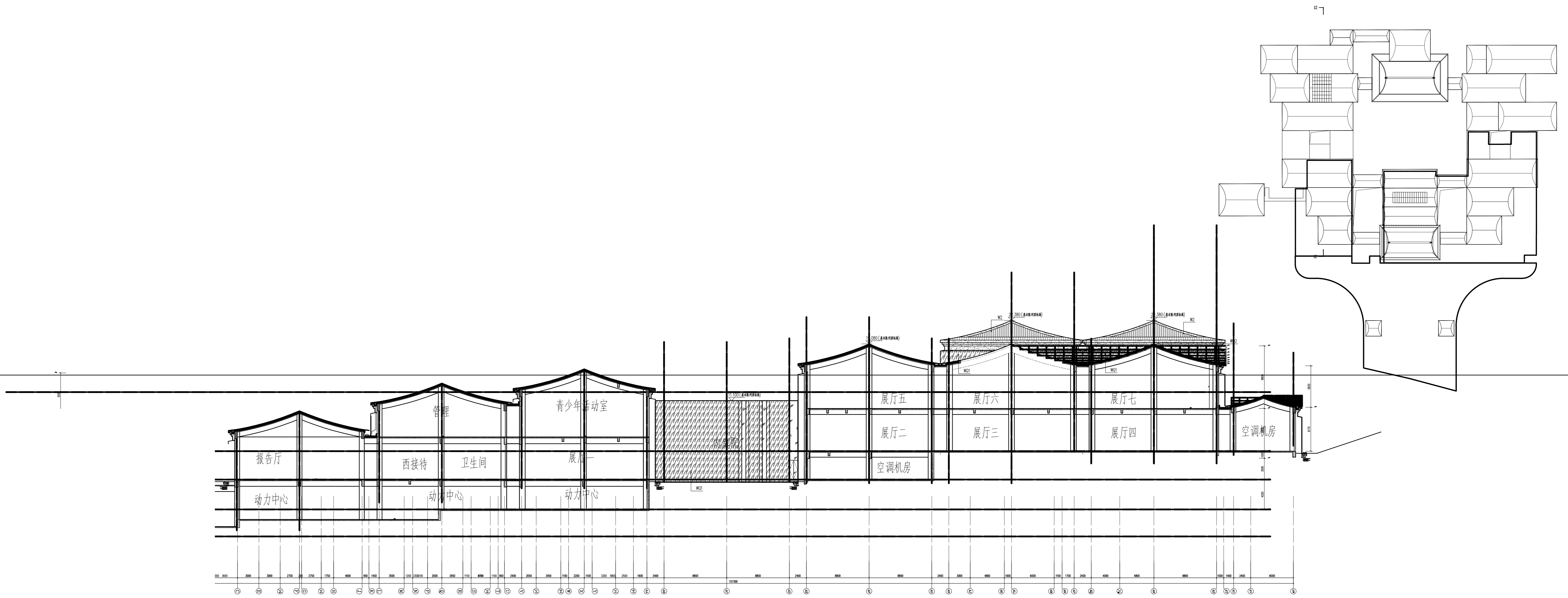
剖面图12 1:150
