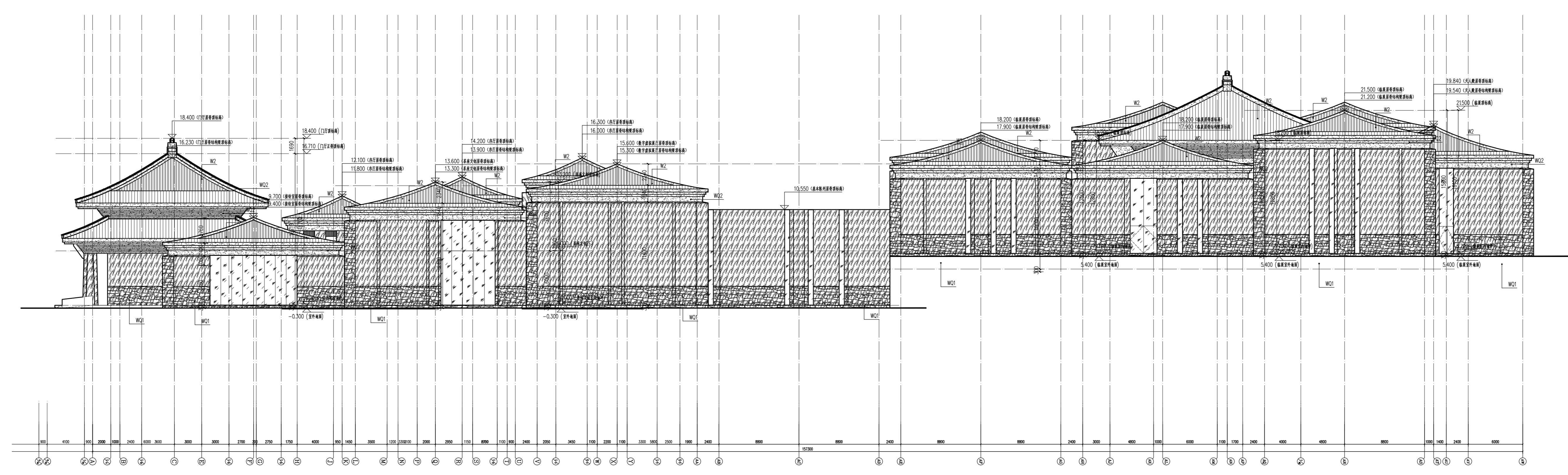
主楼建筑立面全图 1:150
