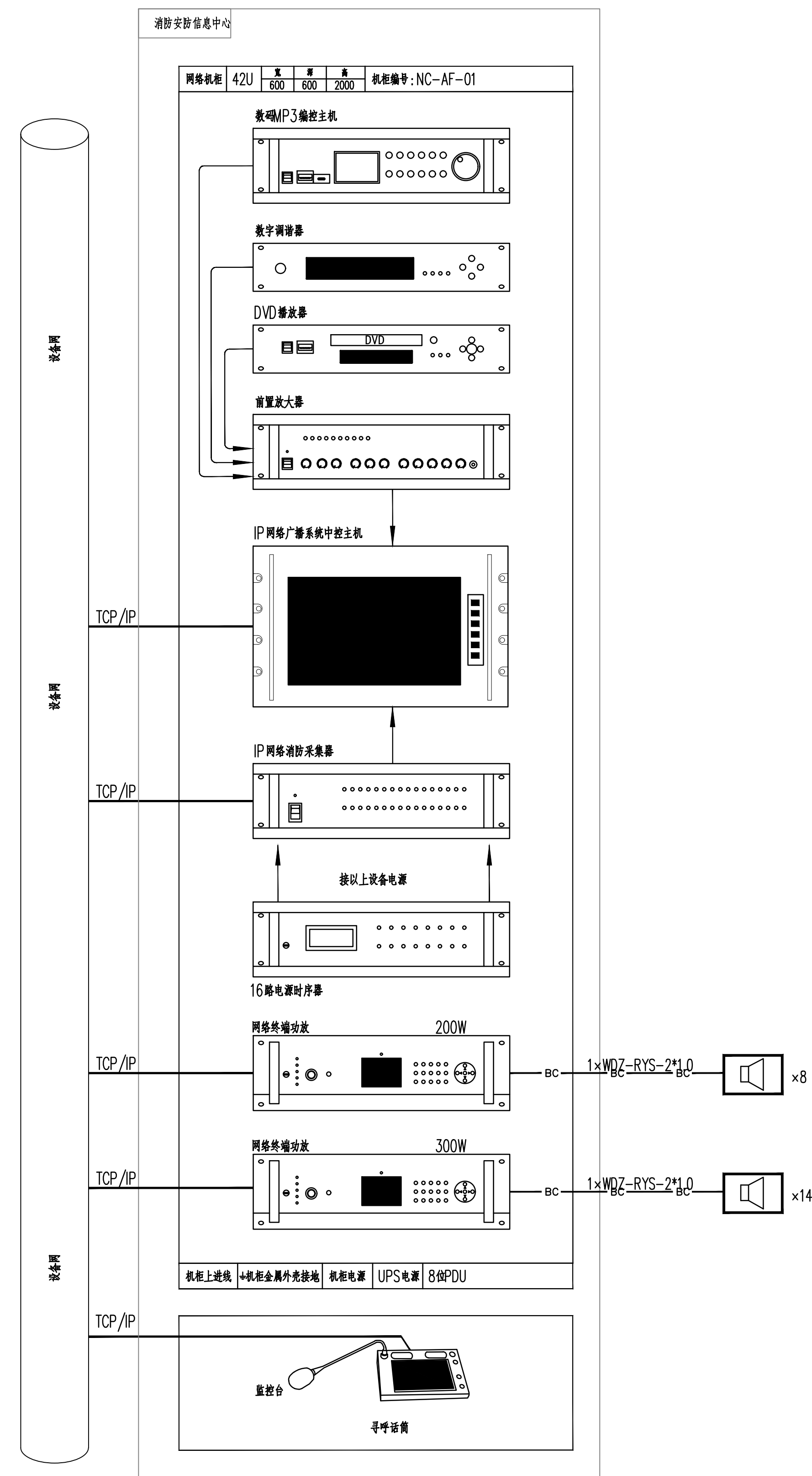
地下公共广播系统图
