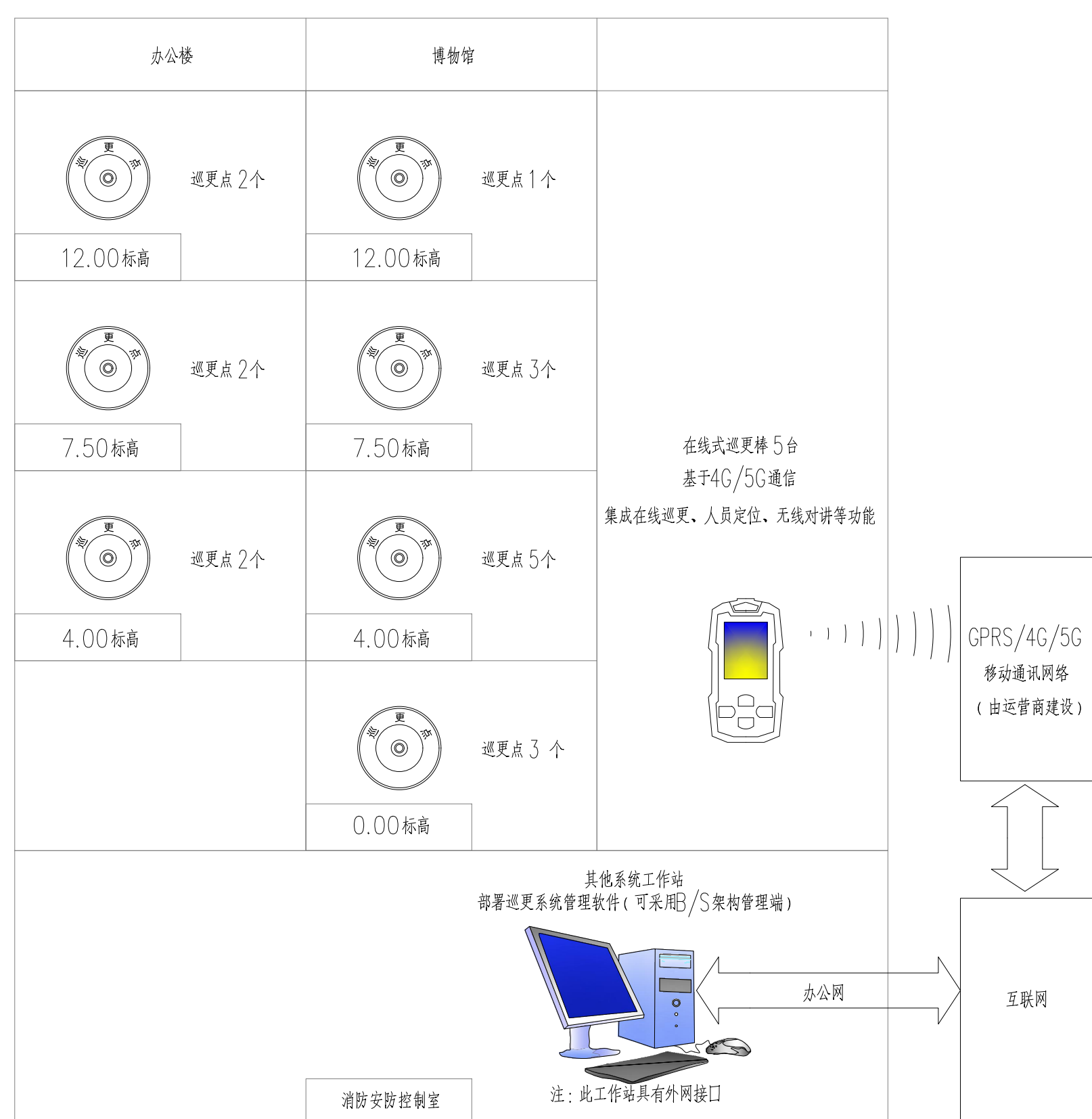
电子巡查(在线式巡更)系统图
