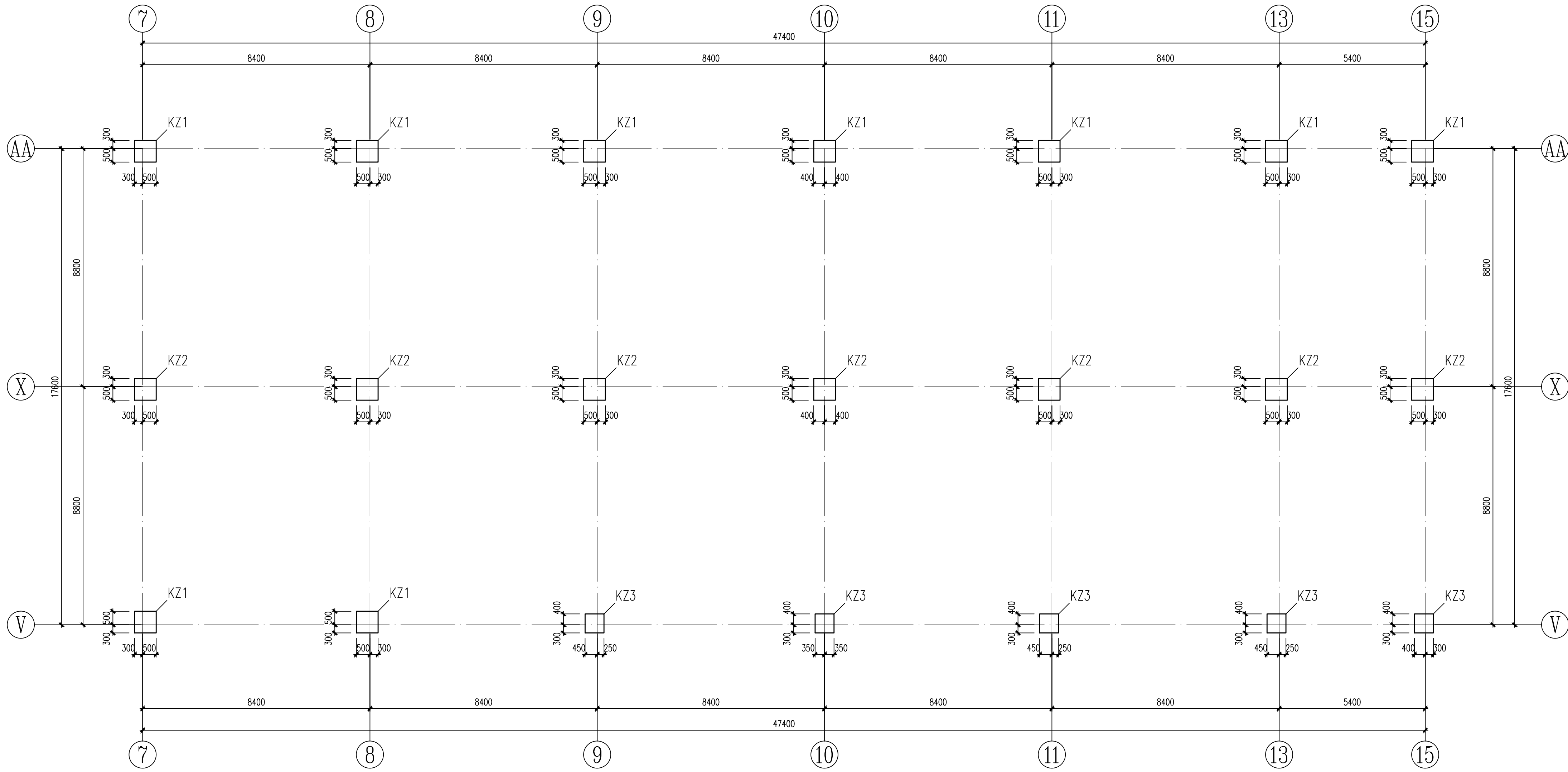
三层柱配筋平面
