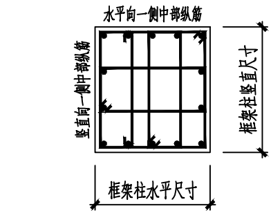
柱配筋示意图 注: 当柱截面中纵筋位置不同时, 应以满足截面配筋率为准
