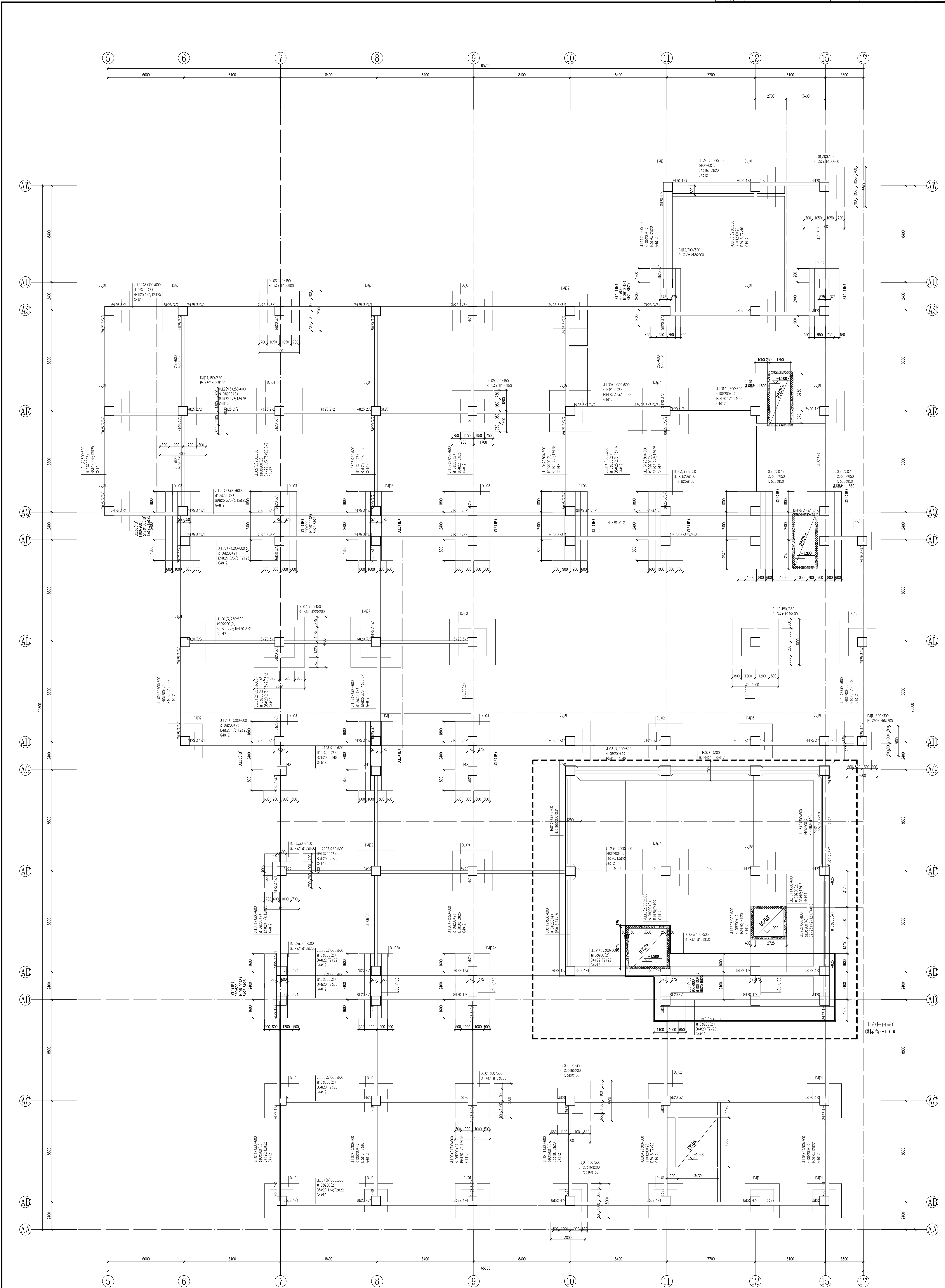
基础结构平面
