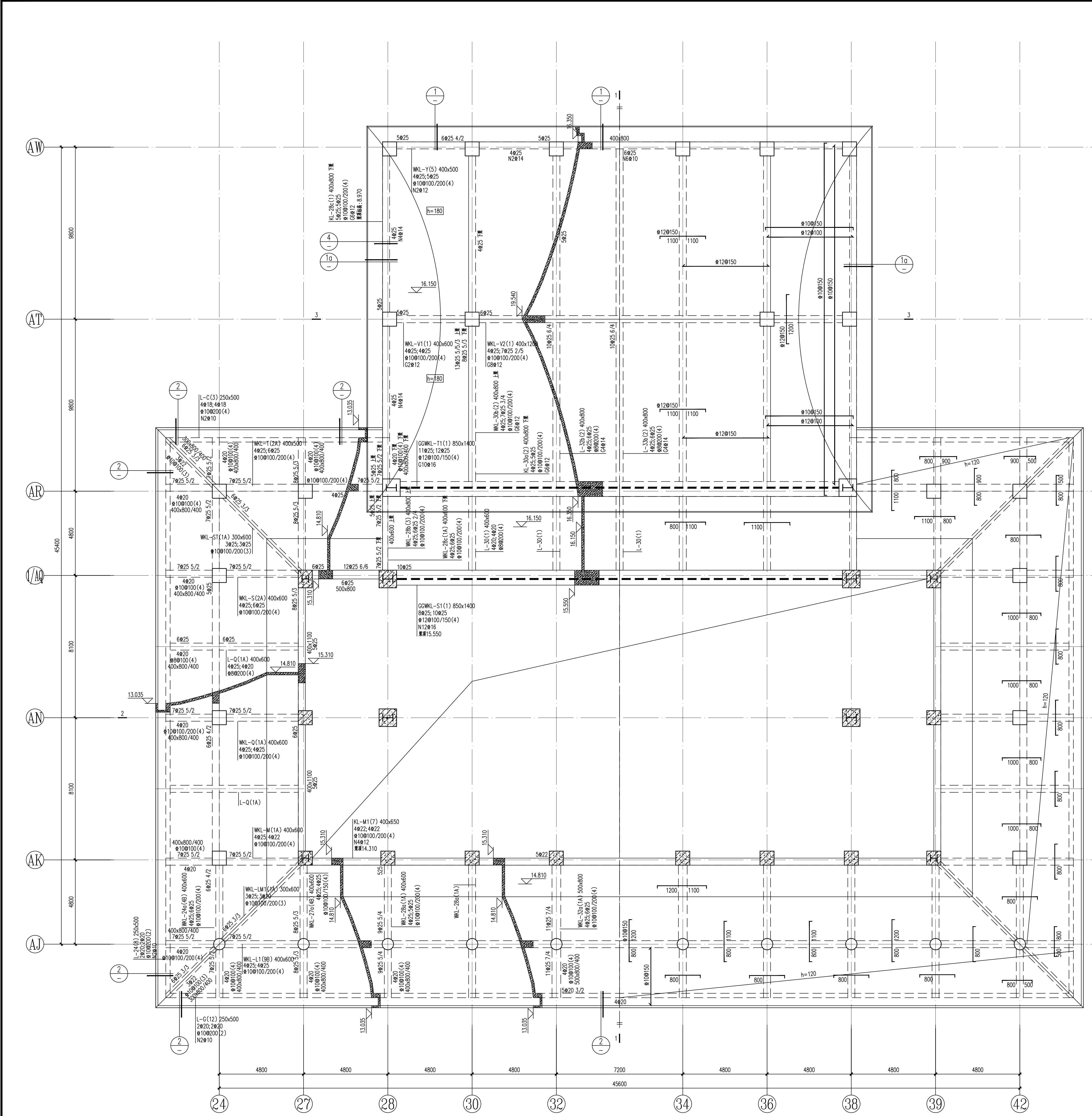
5区局部屋面结构平面
