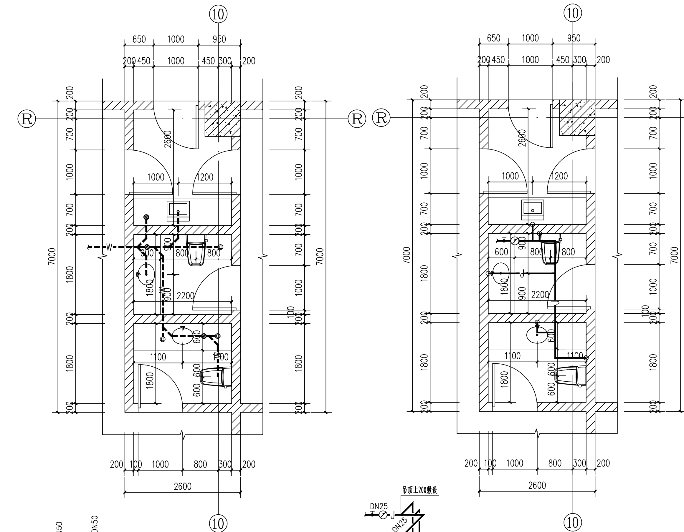
② WSJ2详图 1:50
