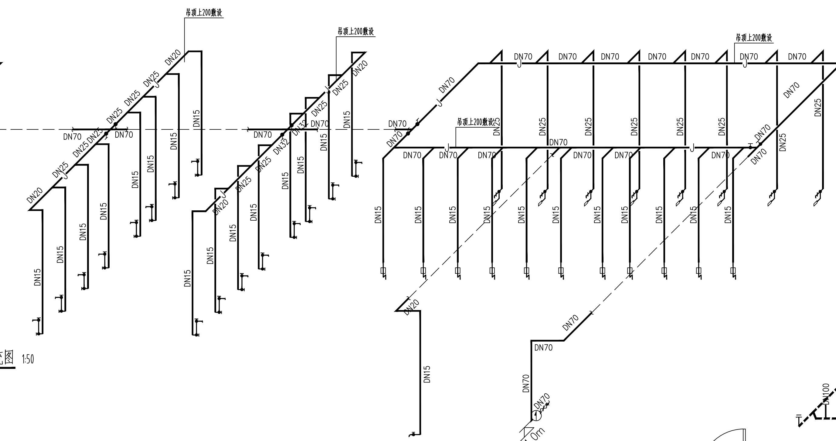
① WSJ1详图 1:50
