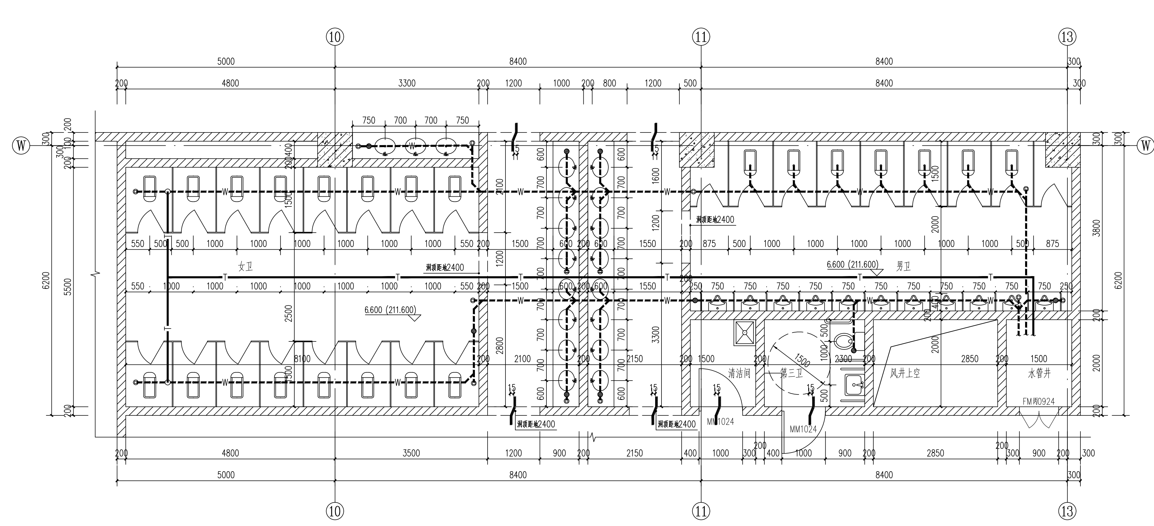
⑤ WSJ5详图 1:50
