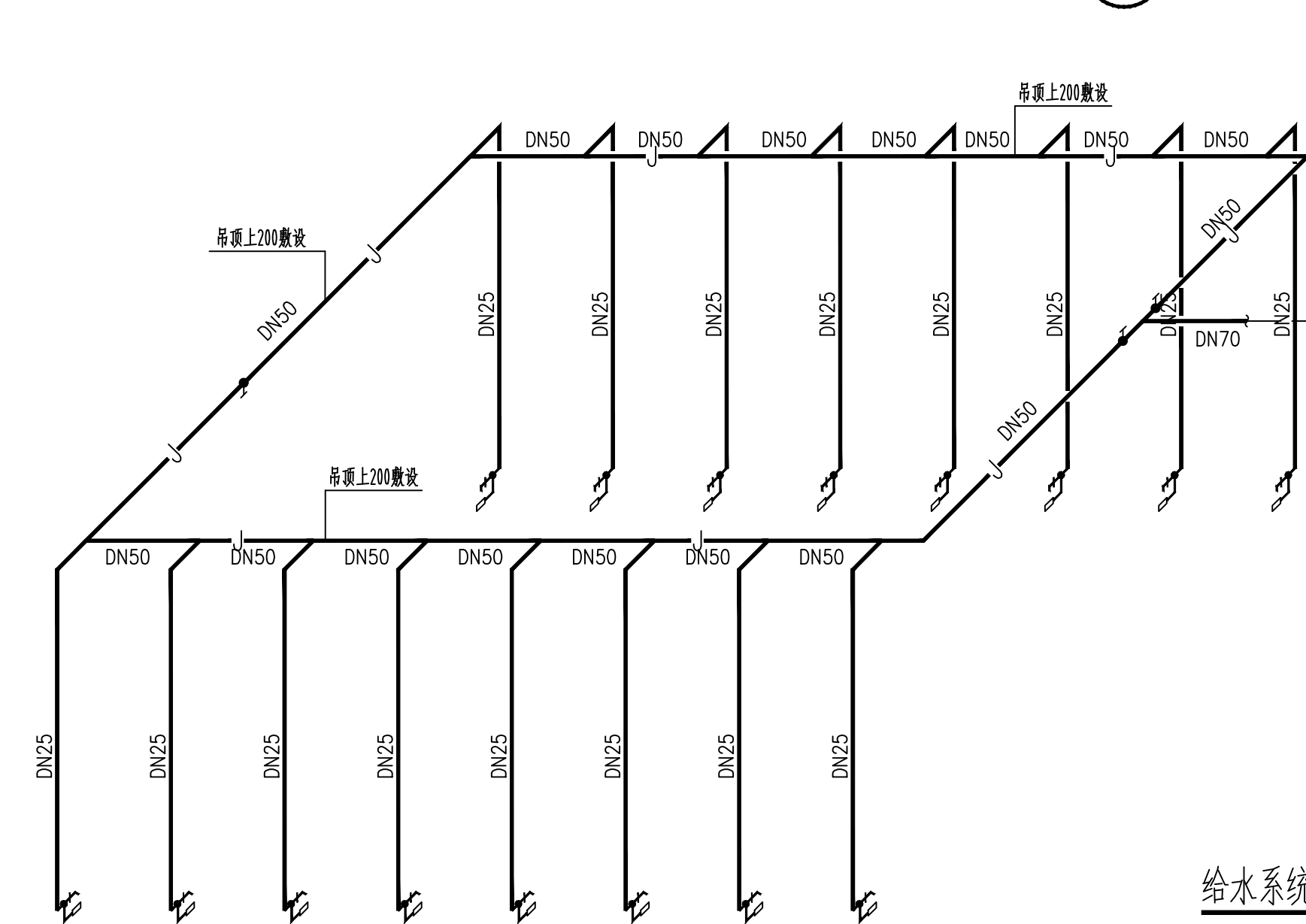
给水系统图 1
