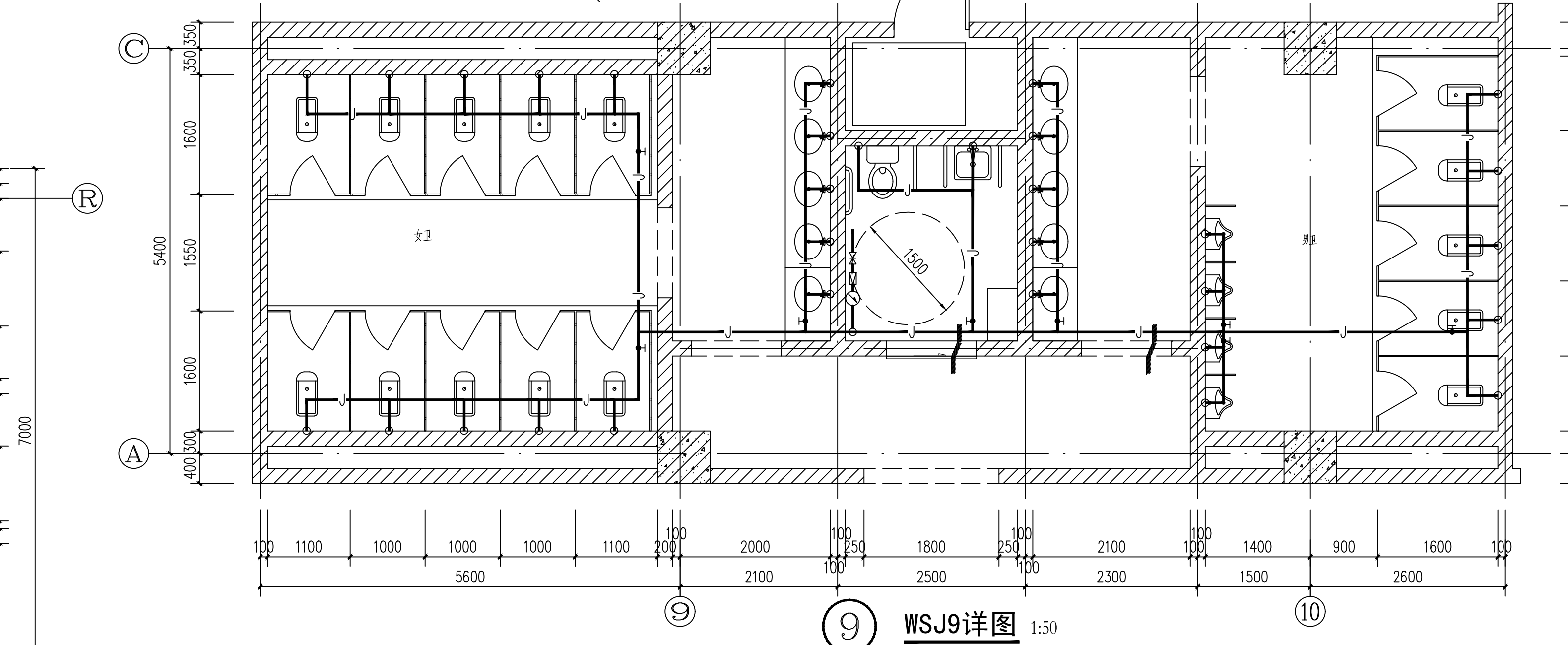
⑨ WSJ9详图 1:50
