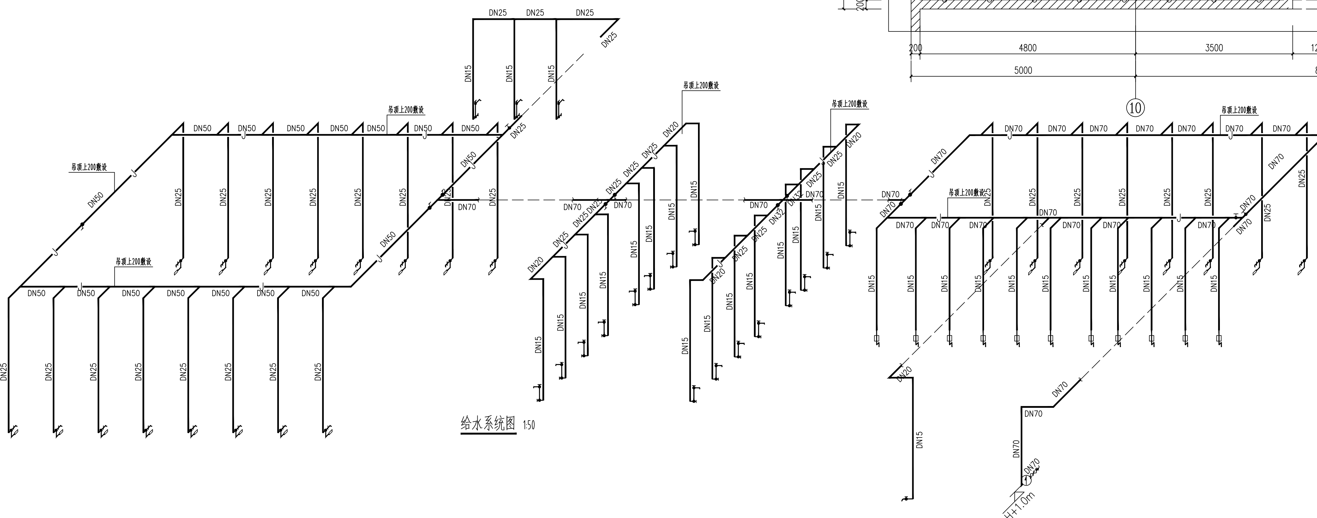
WSJ5详图 1:50
