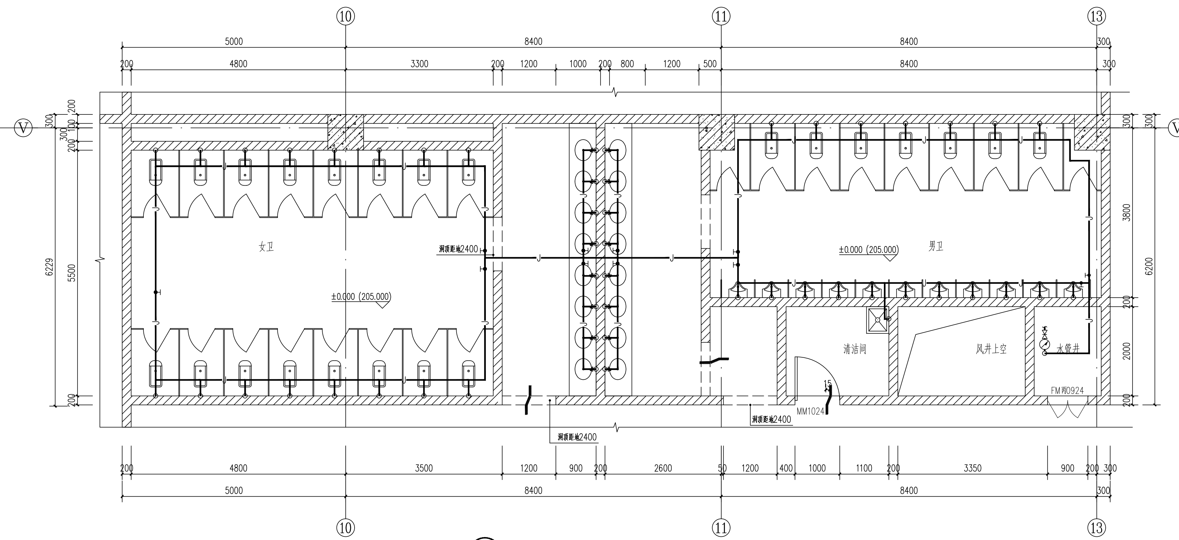
① WSJ1详图 1:50
