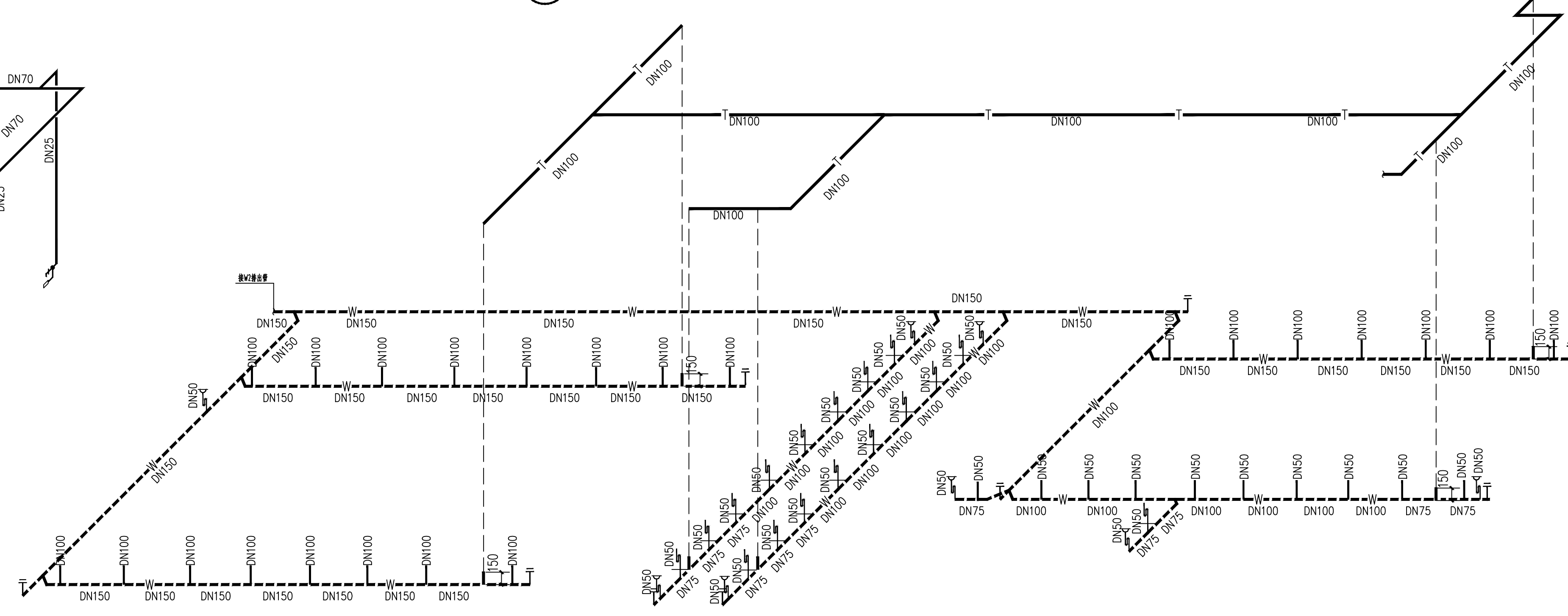
排水系统图 15
