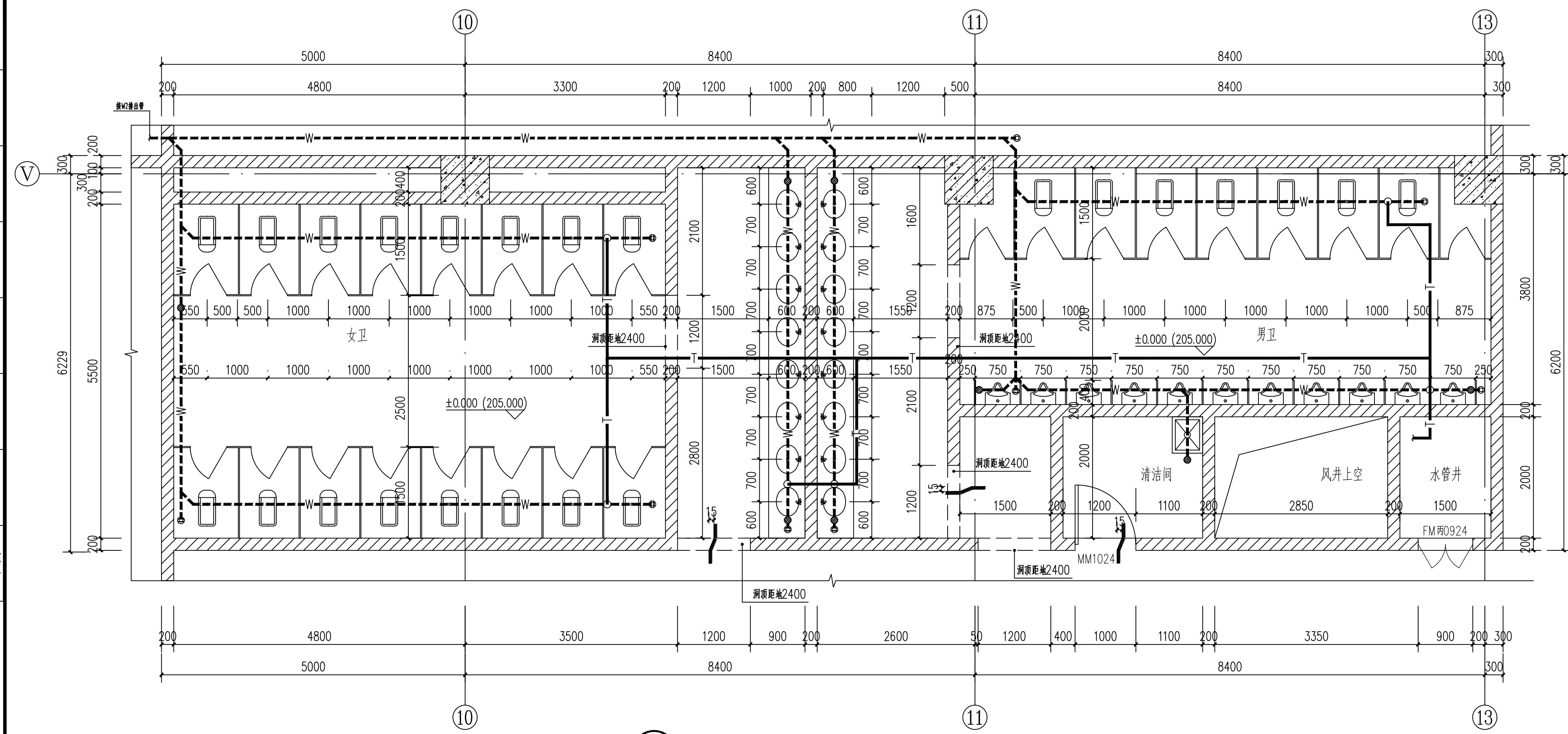
① WSJ1详图 1:50
