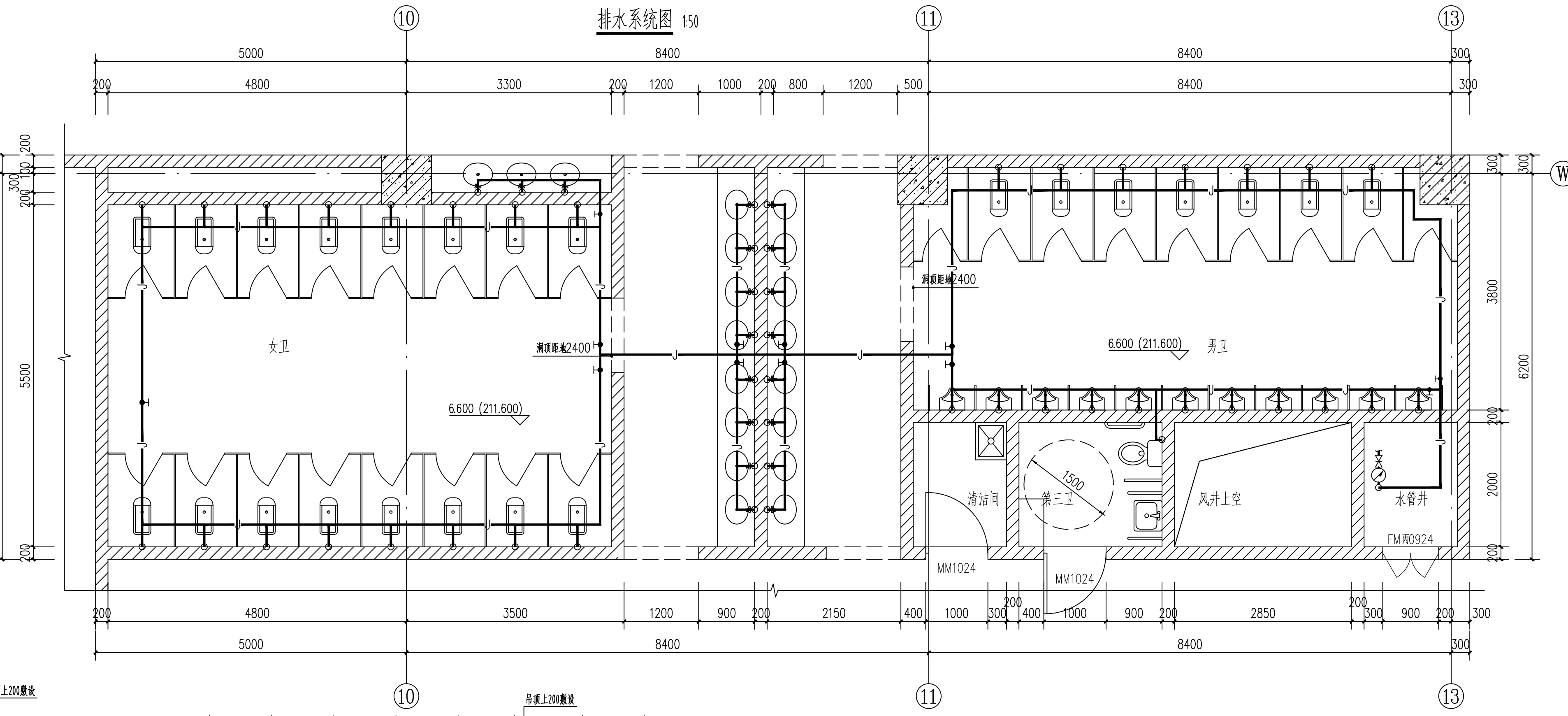
WSJ5详图 1:50
