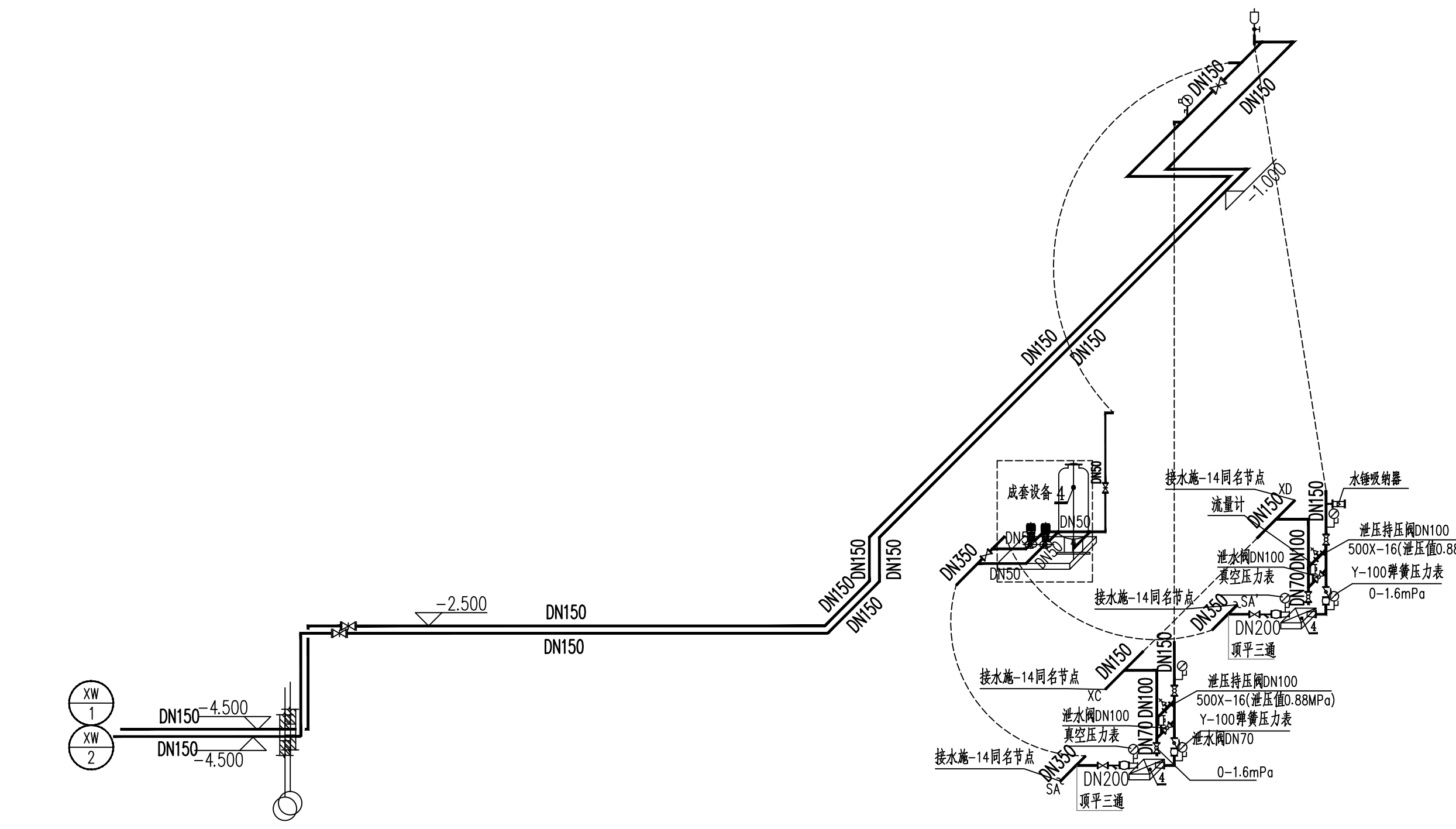
室外消防栓管道系统图 1:50
