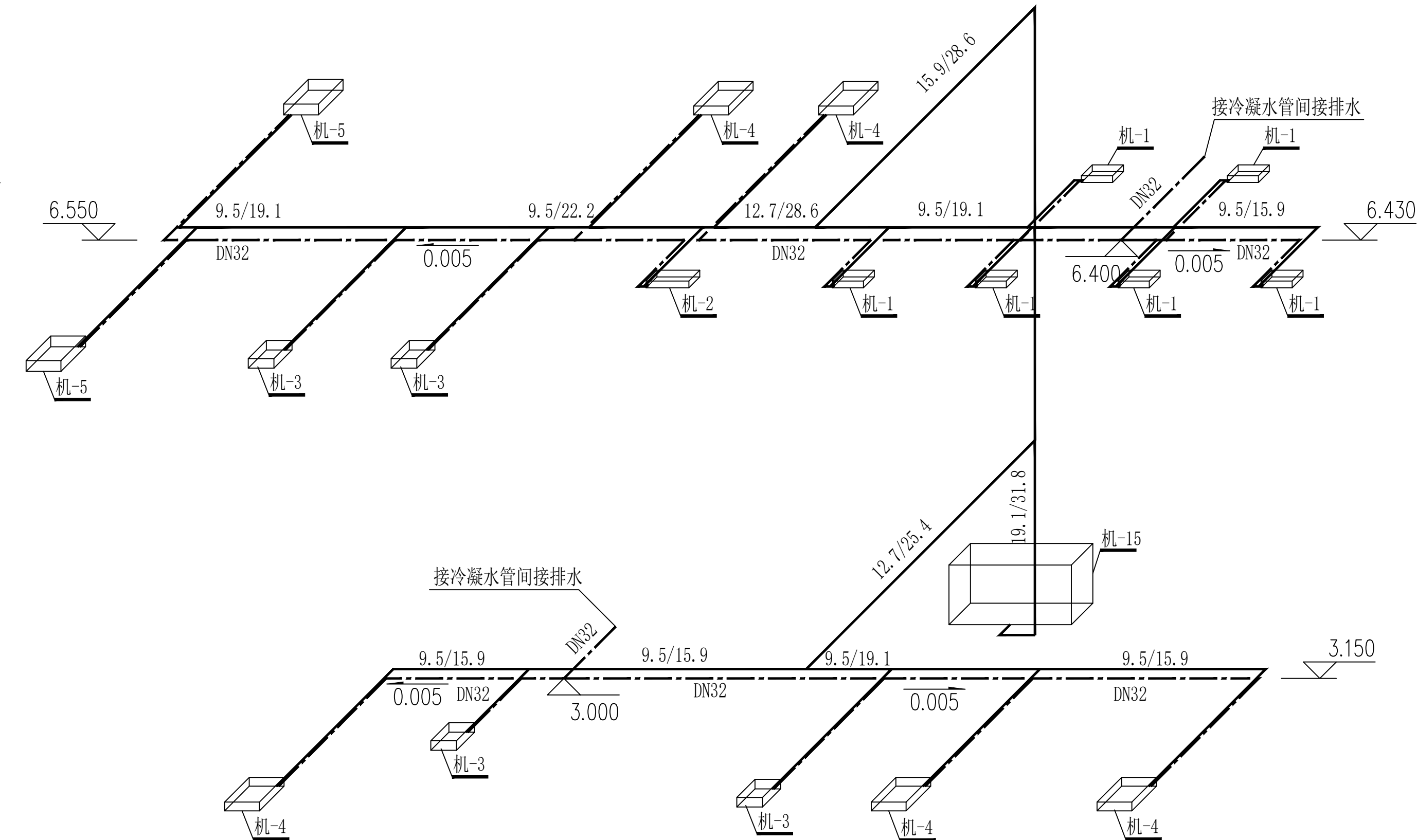
空调系统图
