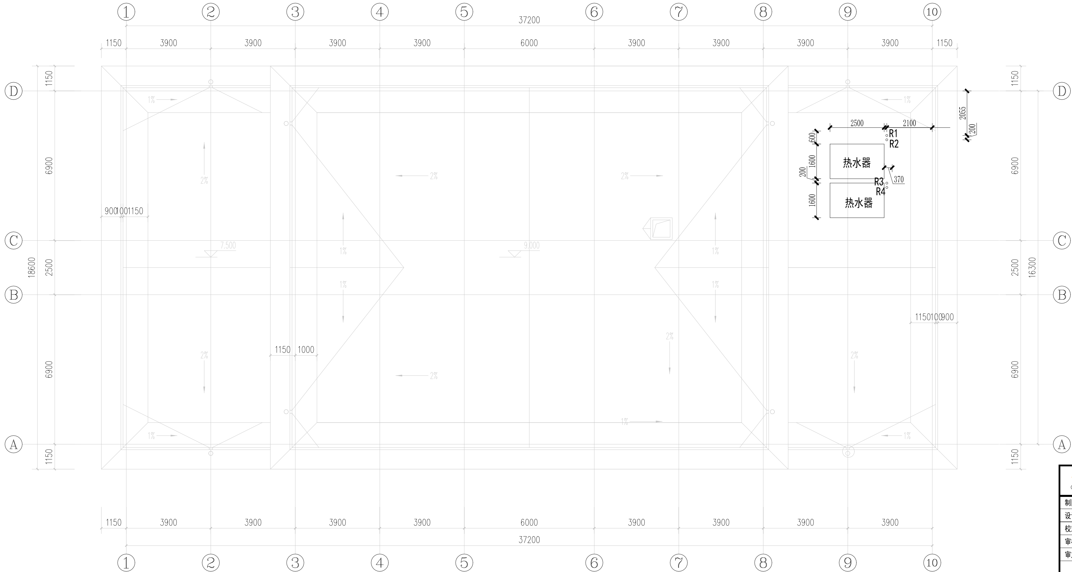
屋面图 1:100
