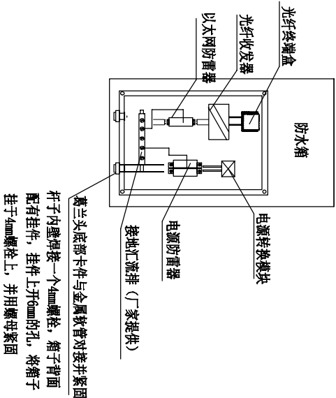
防水箱安装详图
