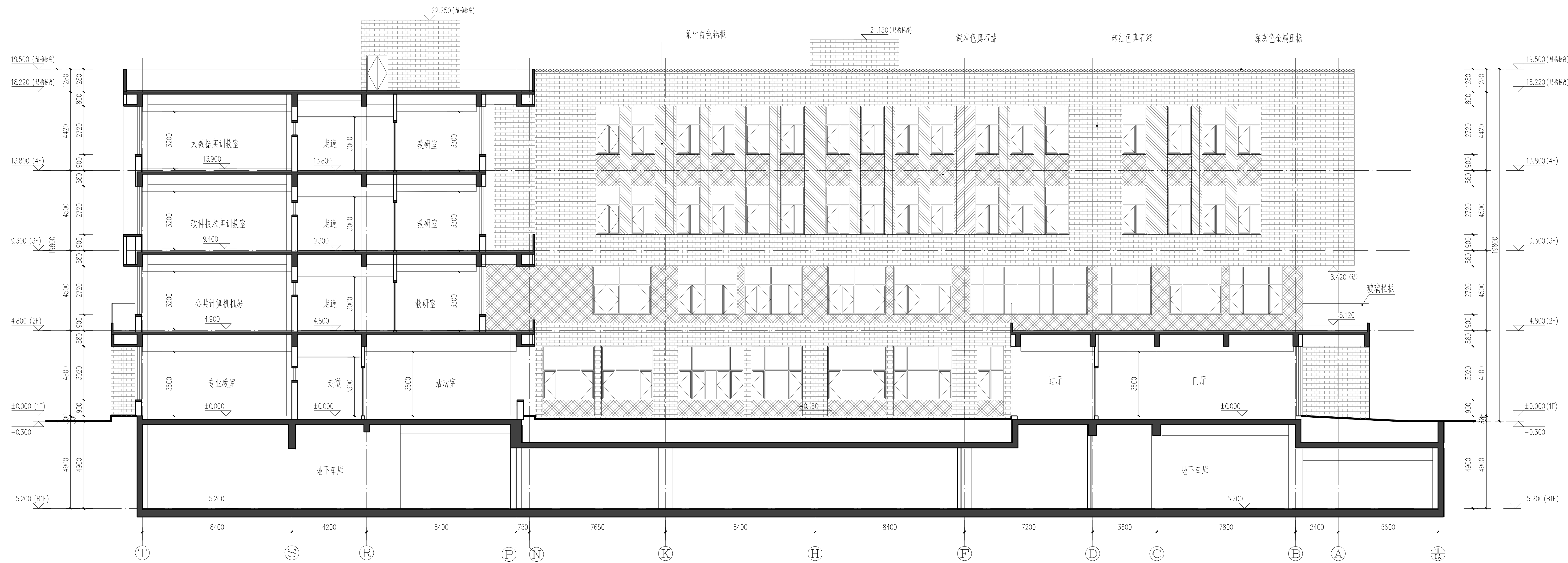
3-3剖面图 1:100
