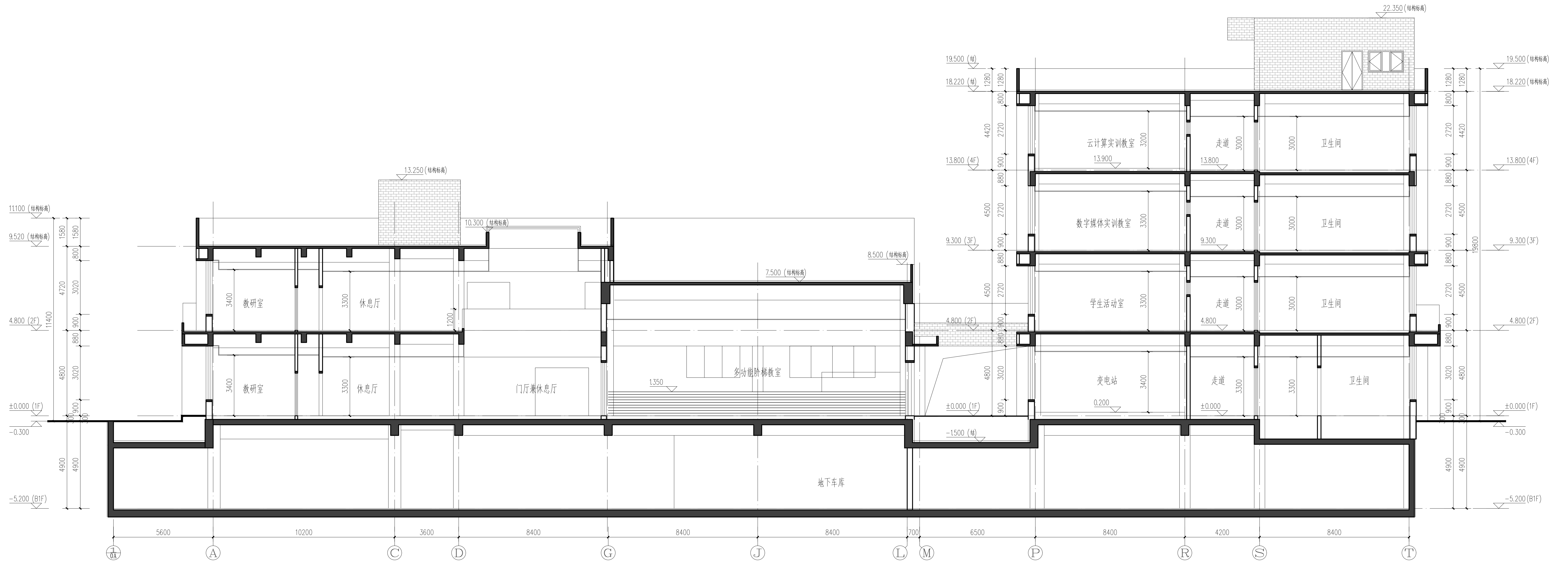
1-1剖面图 1:100
