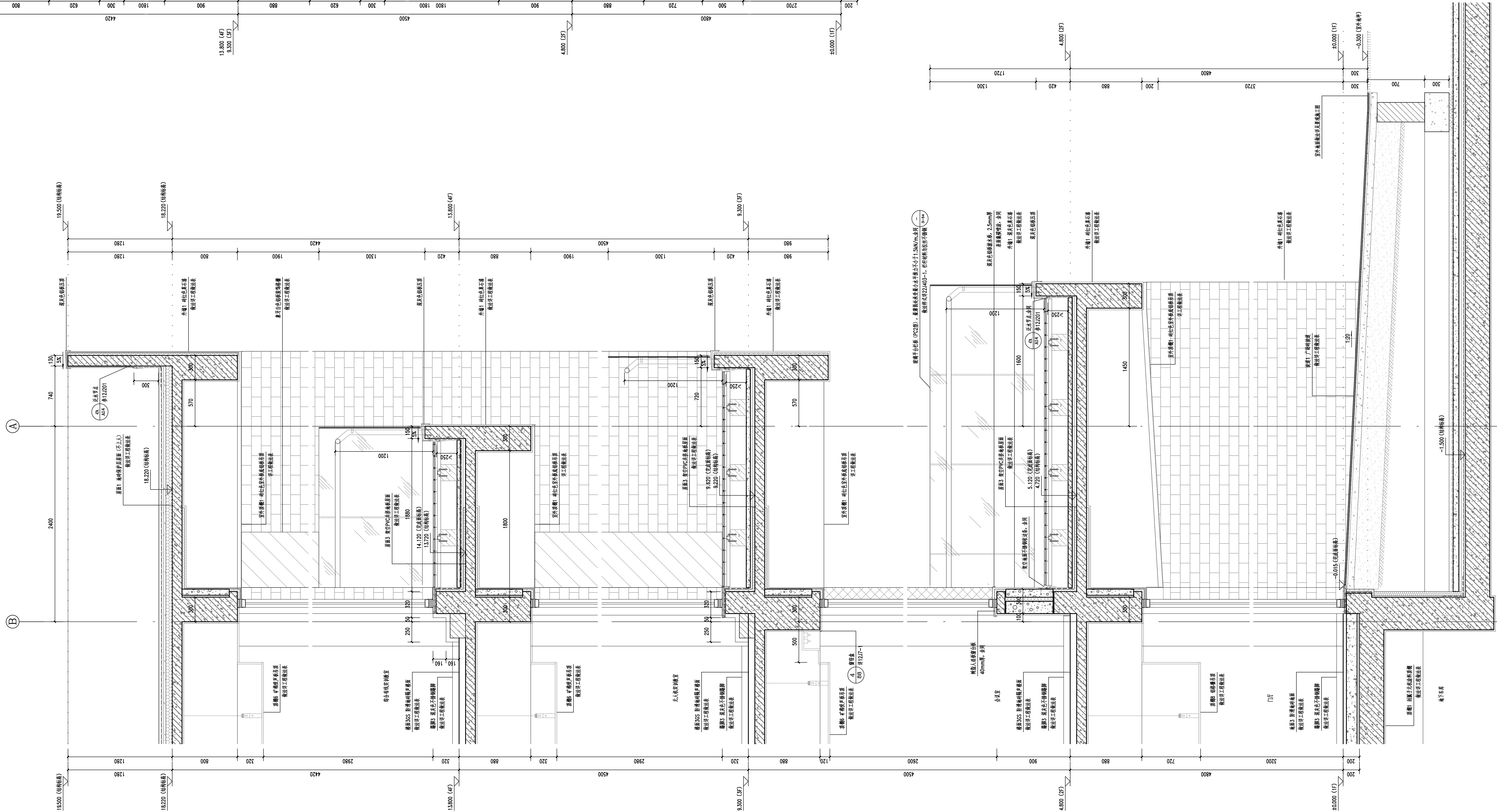
① 外檐详图1 1:20
