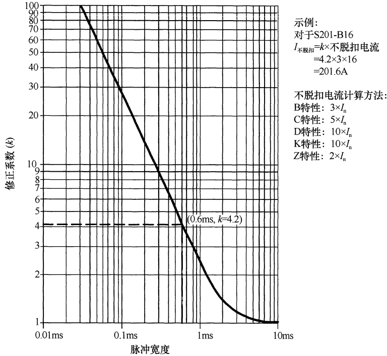
图 6 S201-B16 在毫秒级时间范围的脱扣特性曲线
