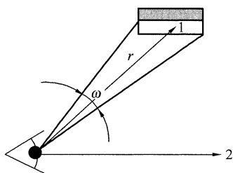
(a) 灯具与观察者关系示意图
