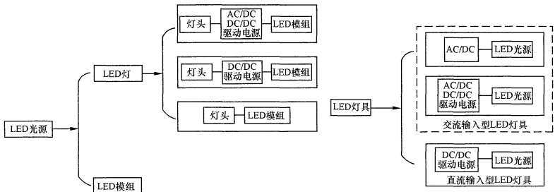
图 1 LED 光源、LED 灯、LED 灯具之间关系图
