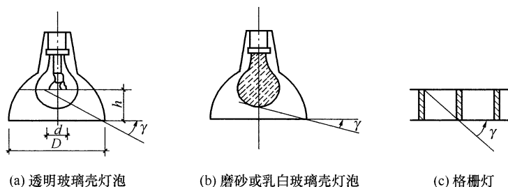
图 4 遮光角示意
