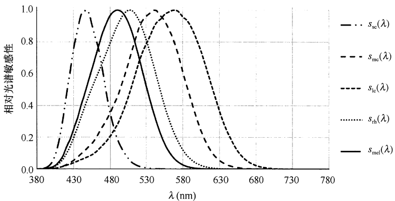
图 2 五种感光蛋白的光谱响应曲线
