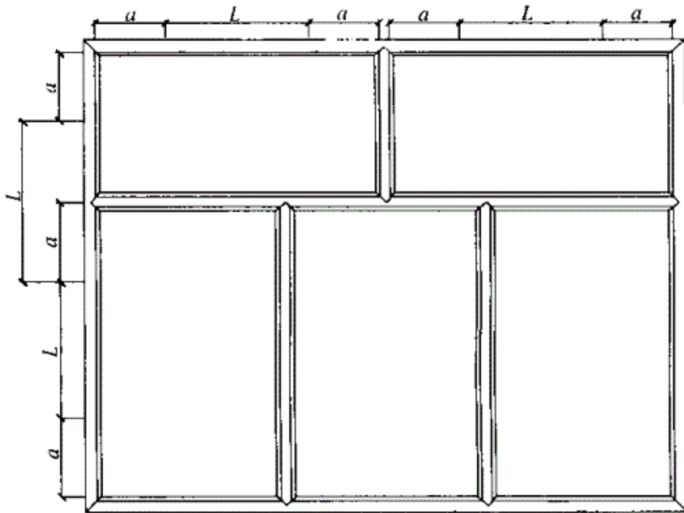
图 6.2.7-2 固定片或膨胀螺钉的安装位置
