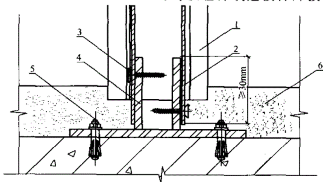
图 6.2.10-1 拼樘料安装节点图 1—拼樘料；2—增强型钢；3—自攻螺钉；4—连接件； 5—膨胀螺钉或射钉；6—伸缩缝填充物
