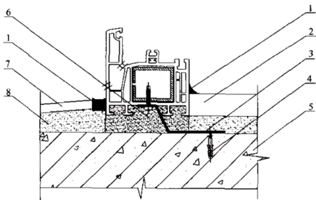
图 6.2.9 窗下框与墙体固定节点图 1—密封胶；2—内窗台板；3 固定片；4—膨胀螺钉； 5—墙体；6—防水砂浆；7—装饰面；8—抹灰层
