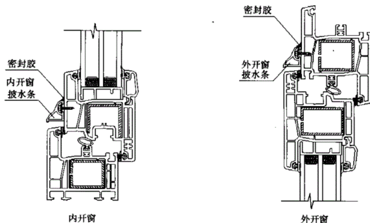
图 3.3.3 披水条安装位置示意图
