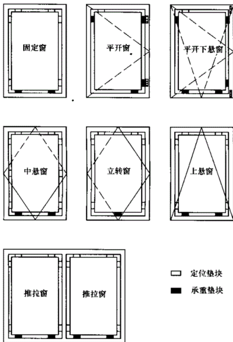
图 6.2.21 承重垫块和定位垫块位置示意图
