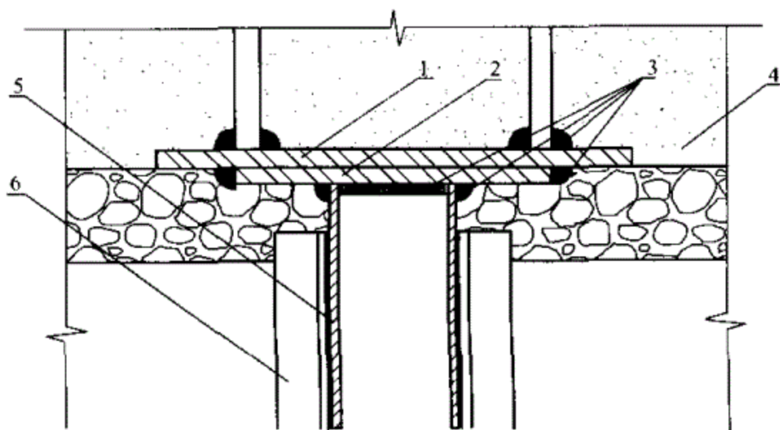
图 6.2.10-2 拼樘料安装节点图
