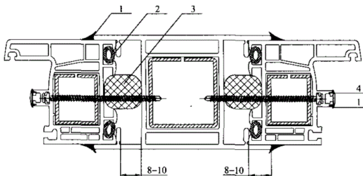
图 6.2.11 拼樘料连接节点图
