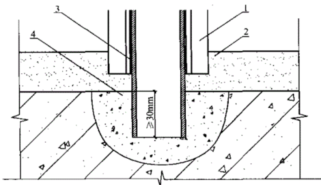
图 6.2.10-3 预留洞口法拼樘料与墙体的固定
