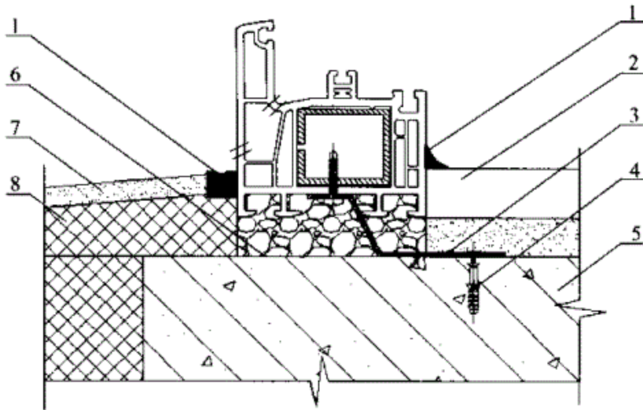
图 6.2.13 外保温墙体窗下框安装节点图
