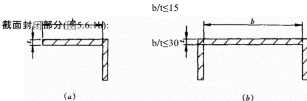
图 5.6.1 截面的厚度
