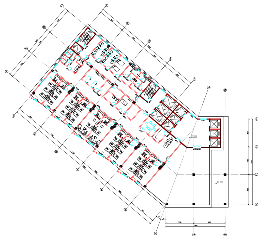
医院住院楼十层平面图 1:500
