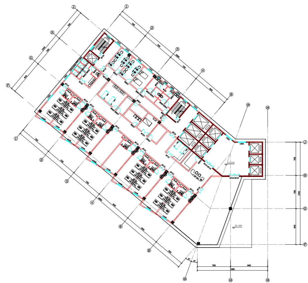
医院住院楼十一层平面图 1:500
