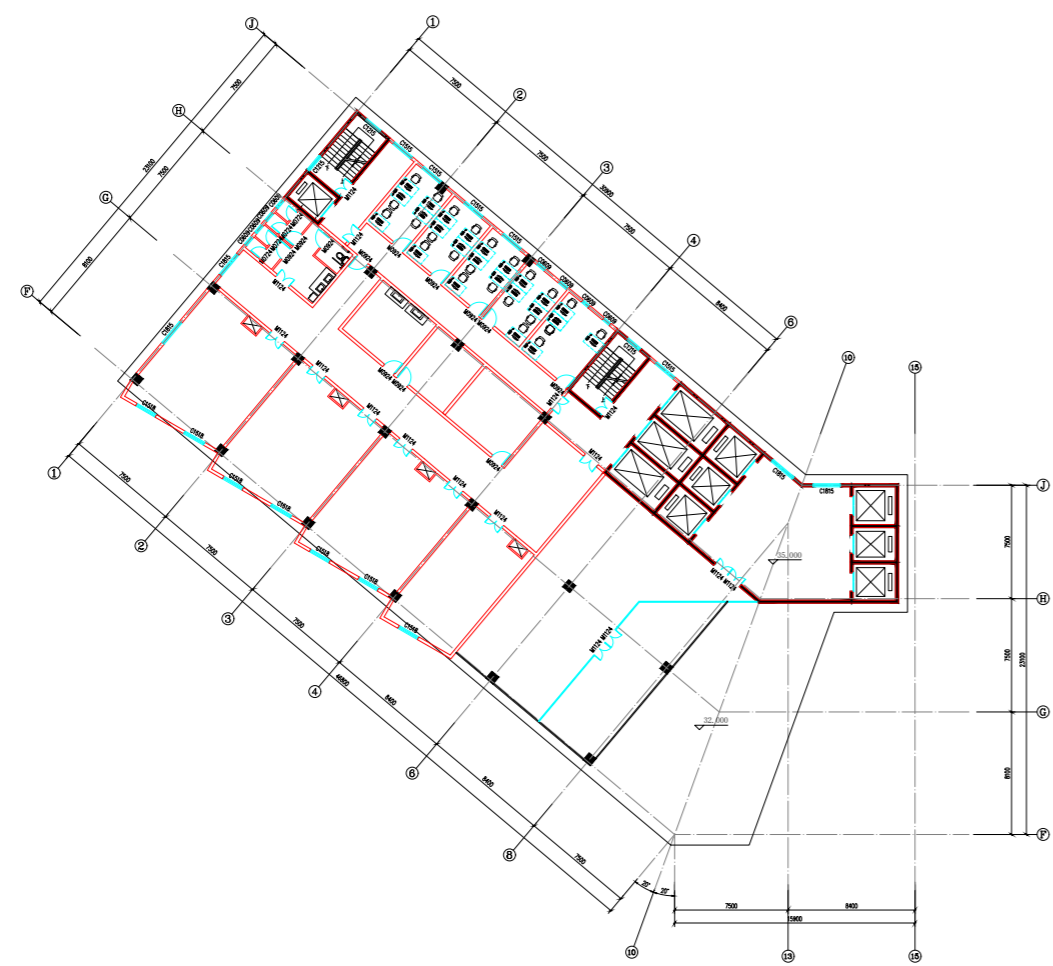
医院住院楼12层平面图 1:500
