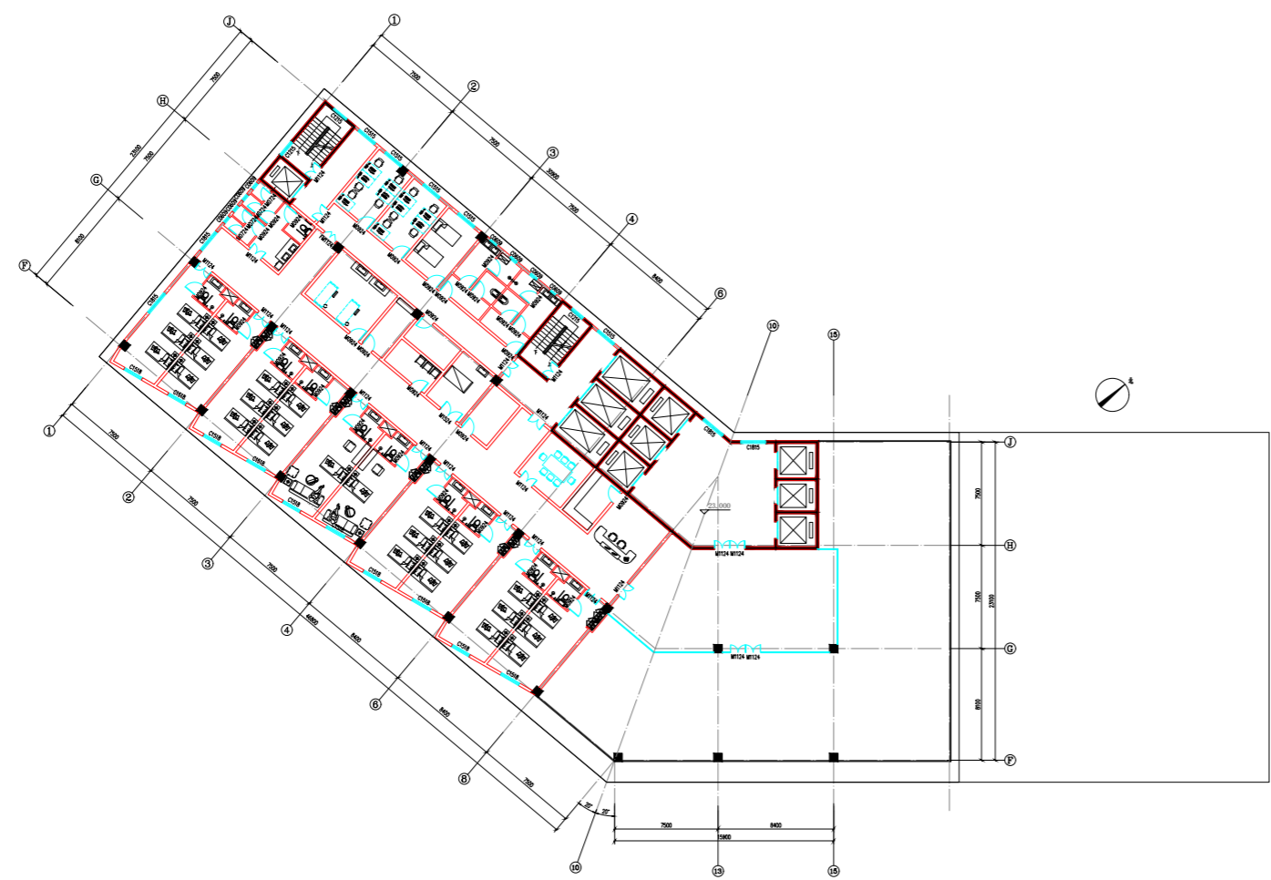
医院住院楼八层平面图 1:500
