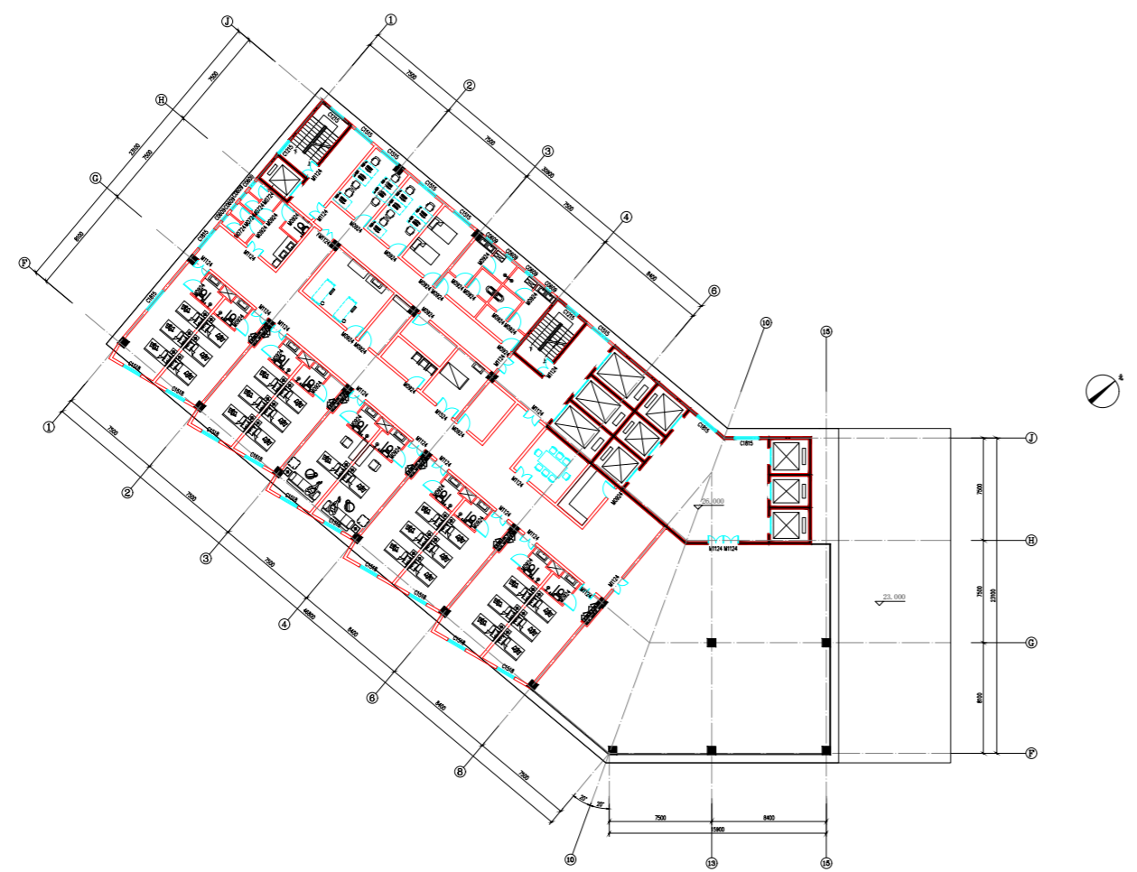
医院住院楼九层平面图 1:500
