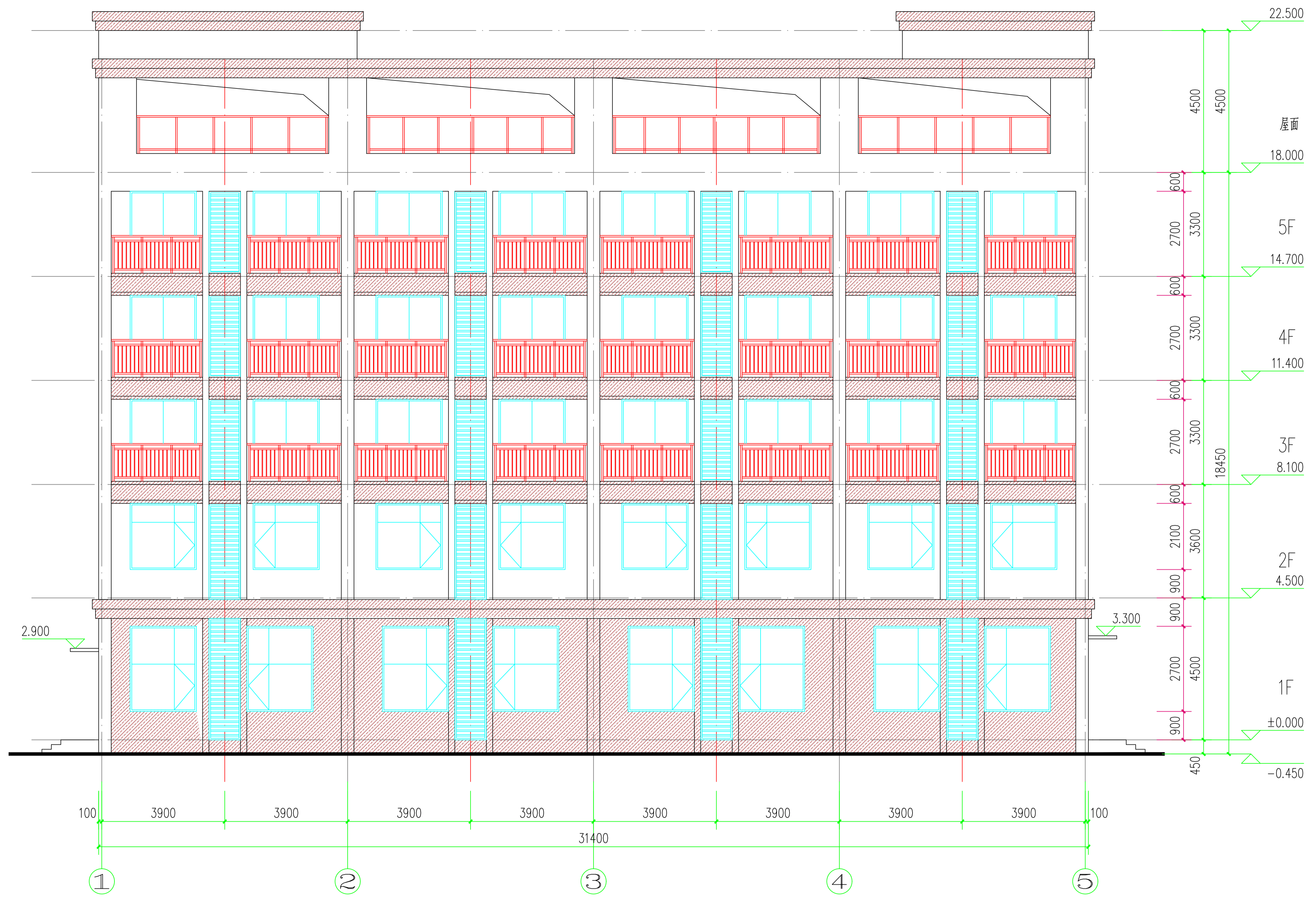
1~轴立面图 1:100
