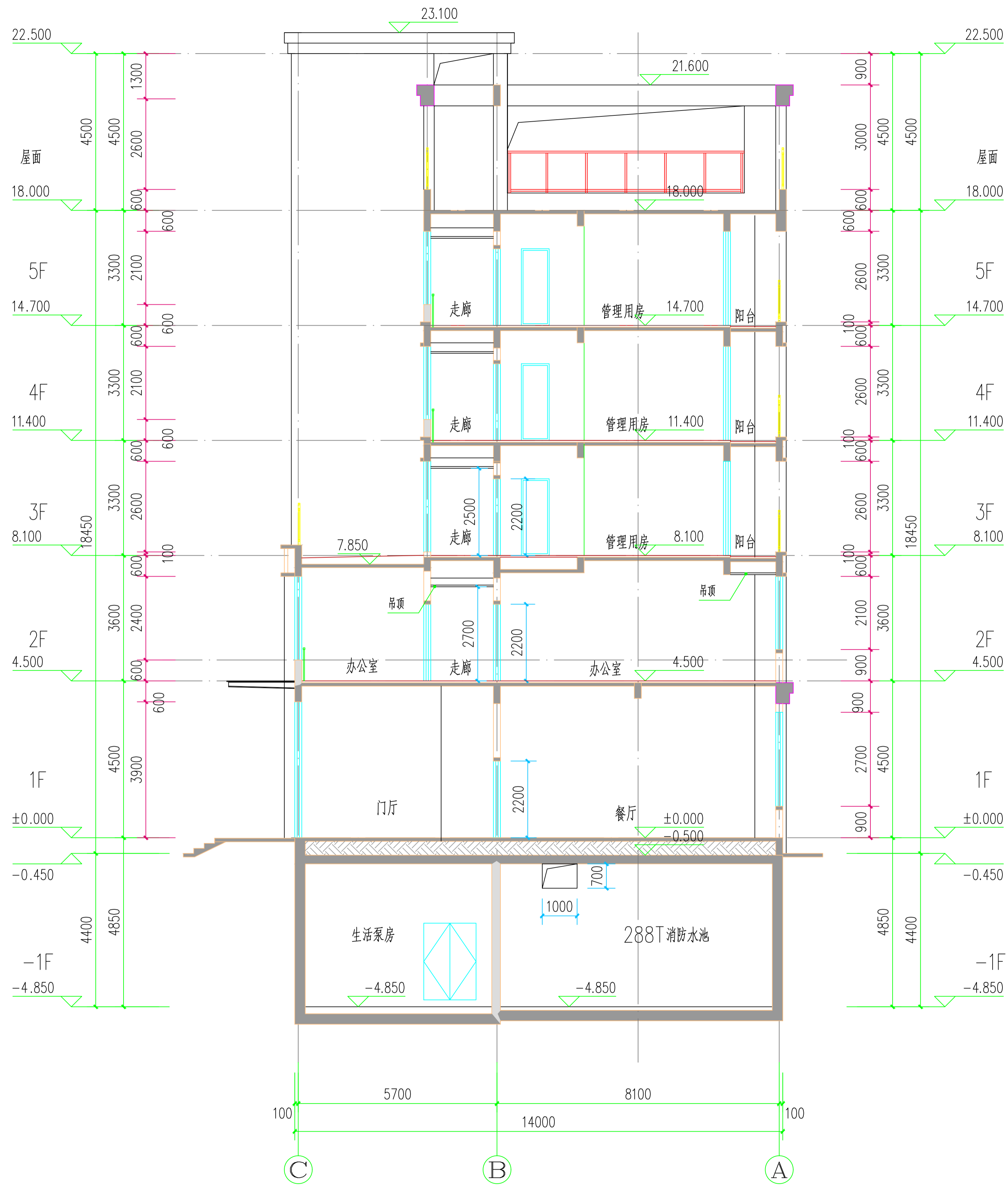
1-剖面图 1:100
