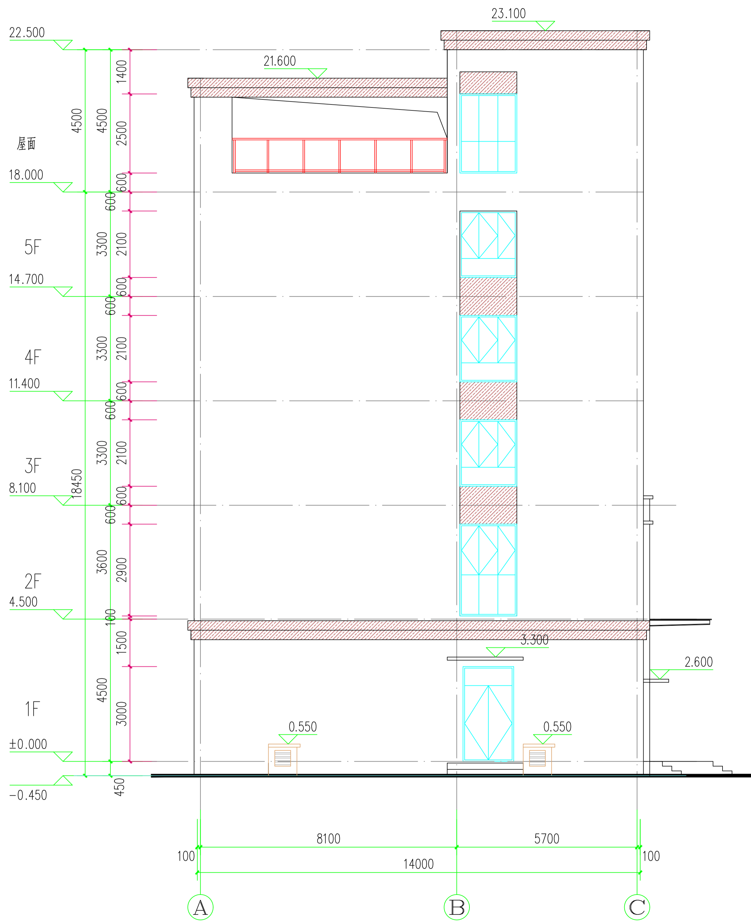
A~轴立面图 1:100
