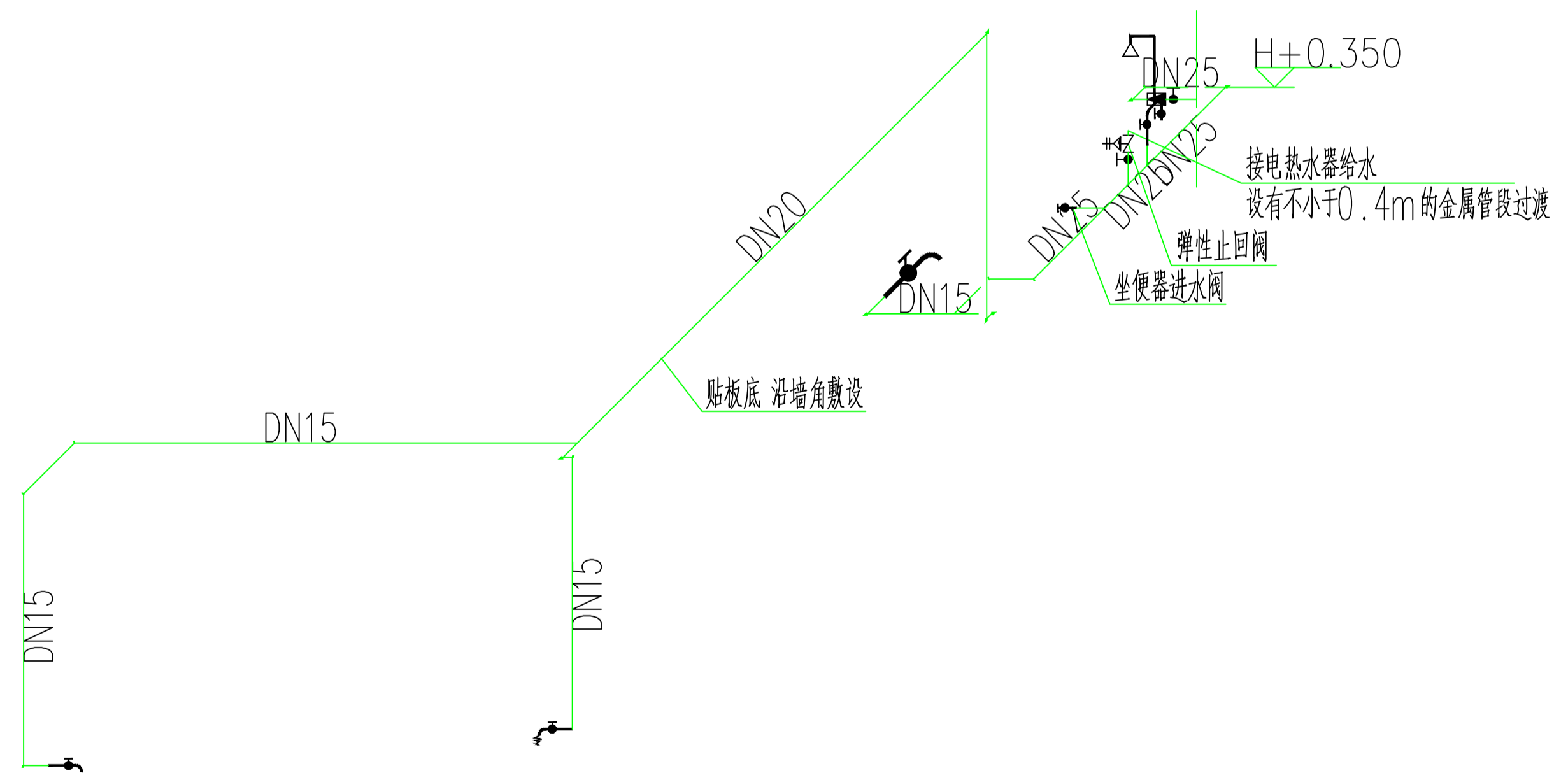
管理用房给水放大图 1:50
