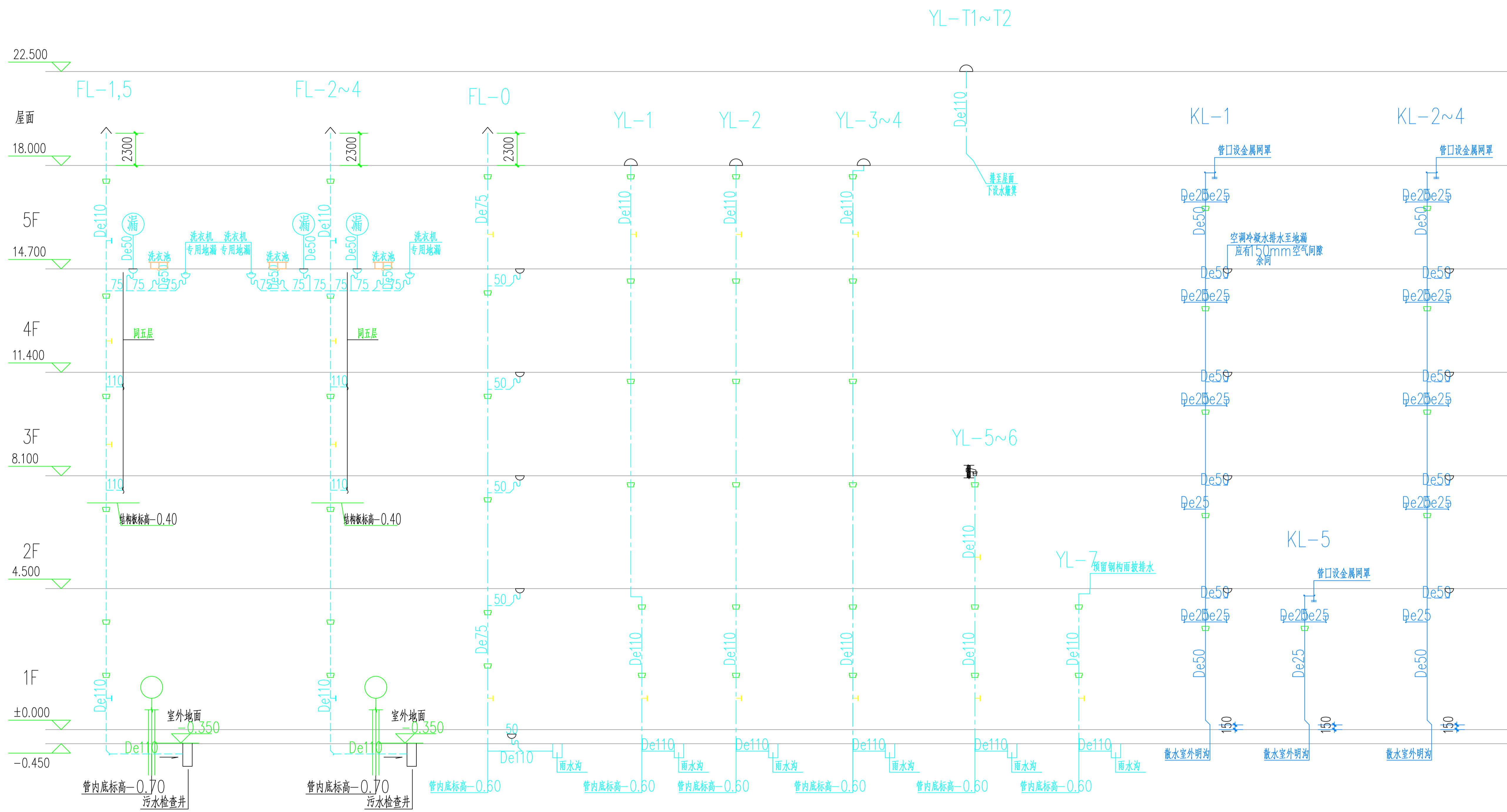
冷凝水系统原理图
