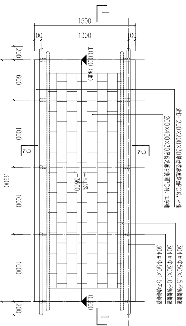
1 残疾人坡道平面图 1:25
