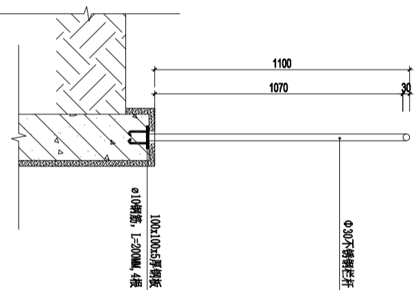
6 不锈钢栏杆剖面图 SCALE 1:15
