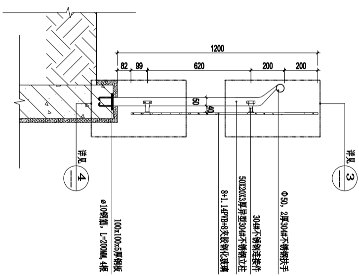
2 玻璃栏杆剖面图 SCALE 1:15
