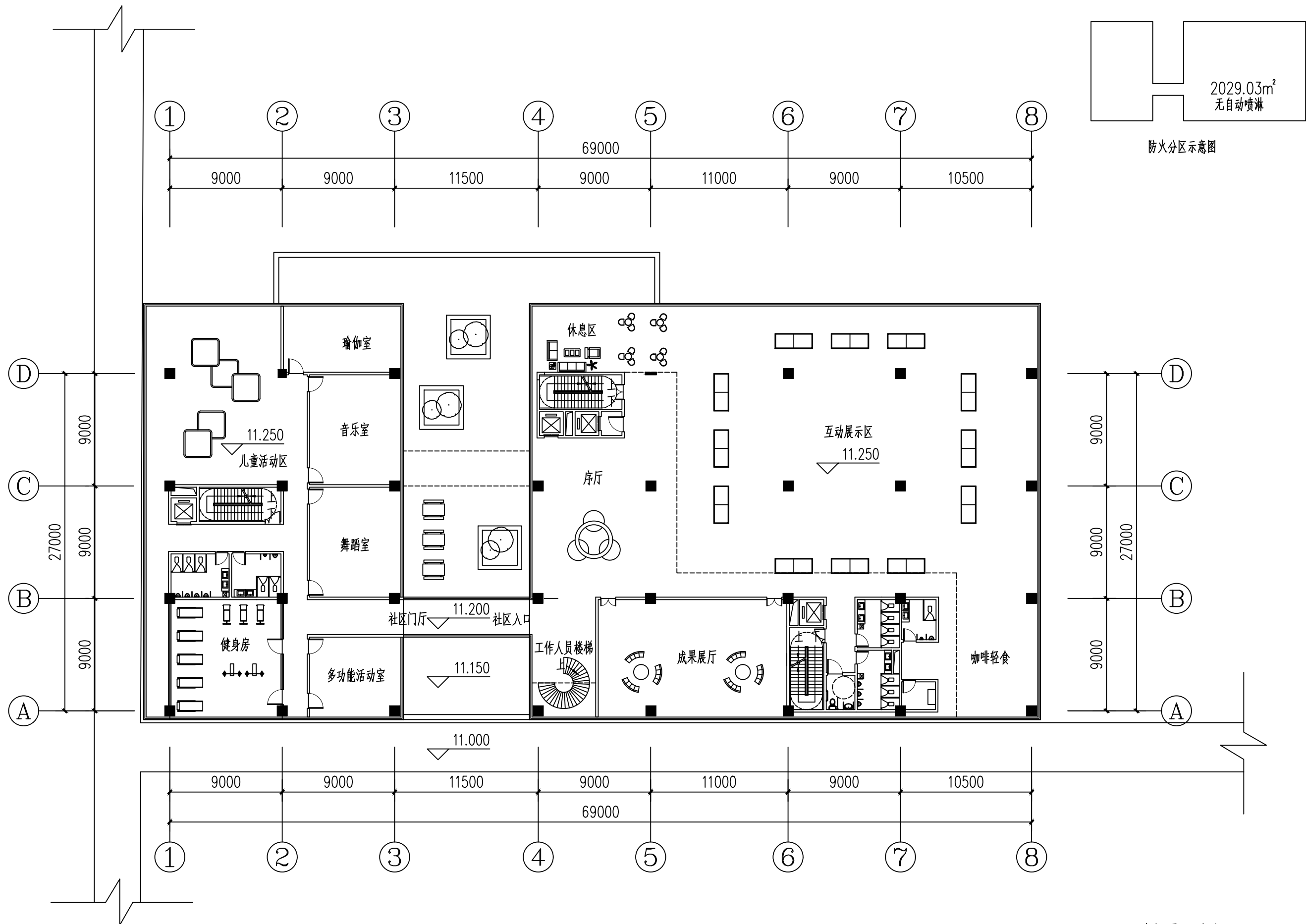
三层平面图 1:300
