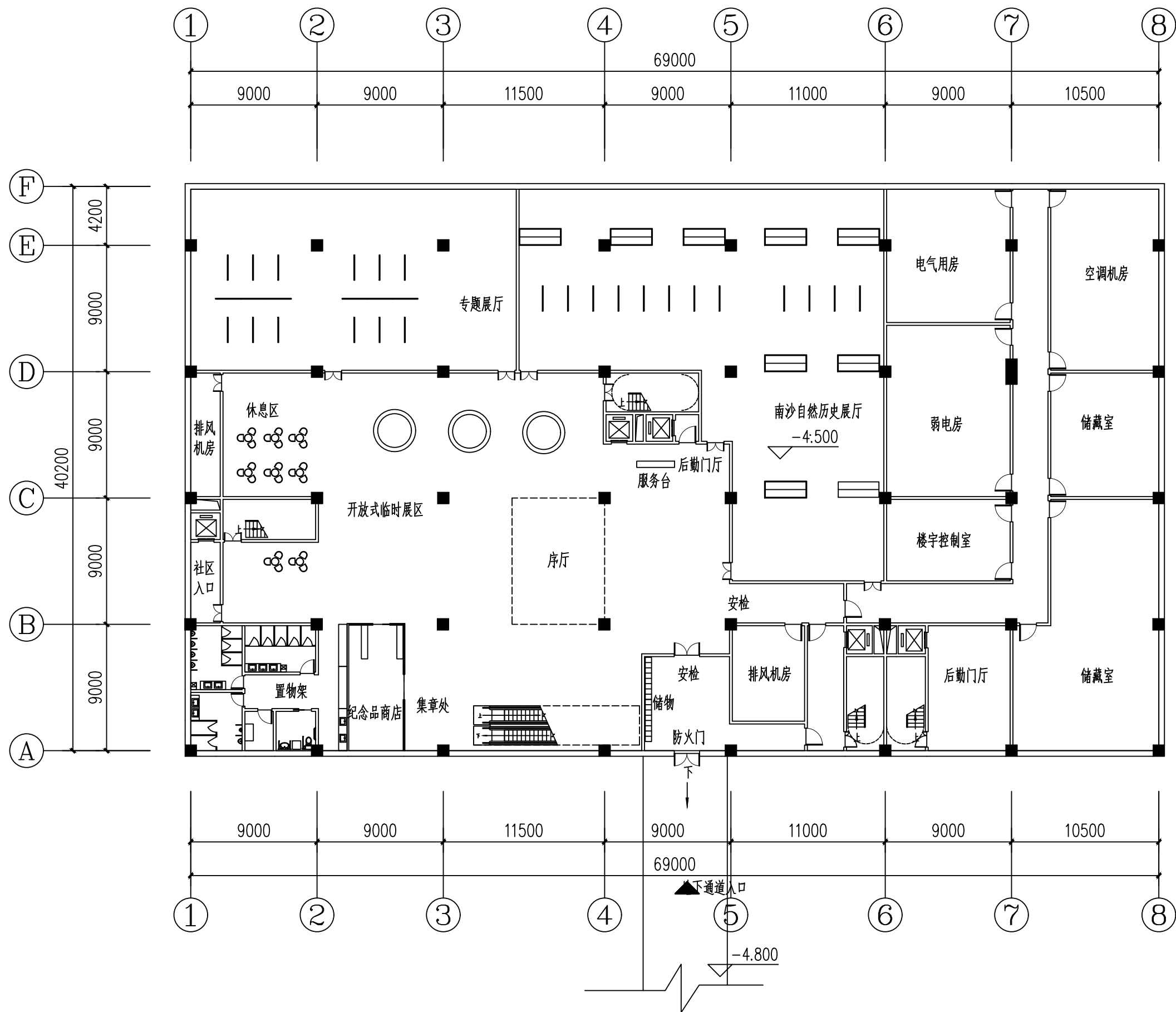
地下一层平面图 1:300
