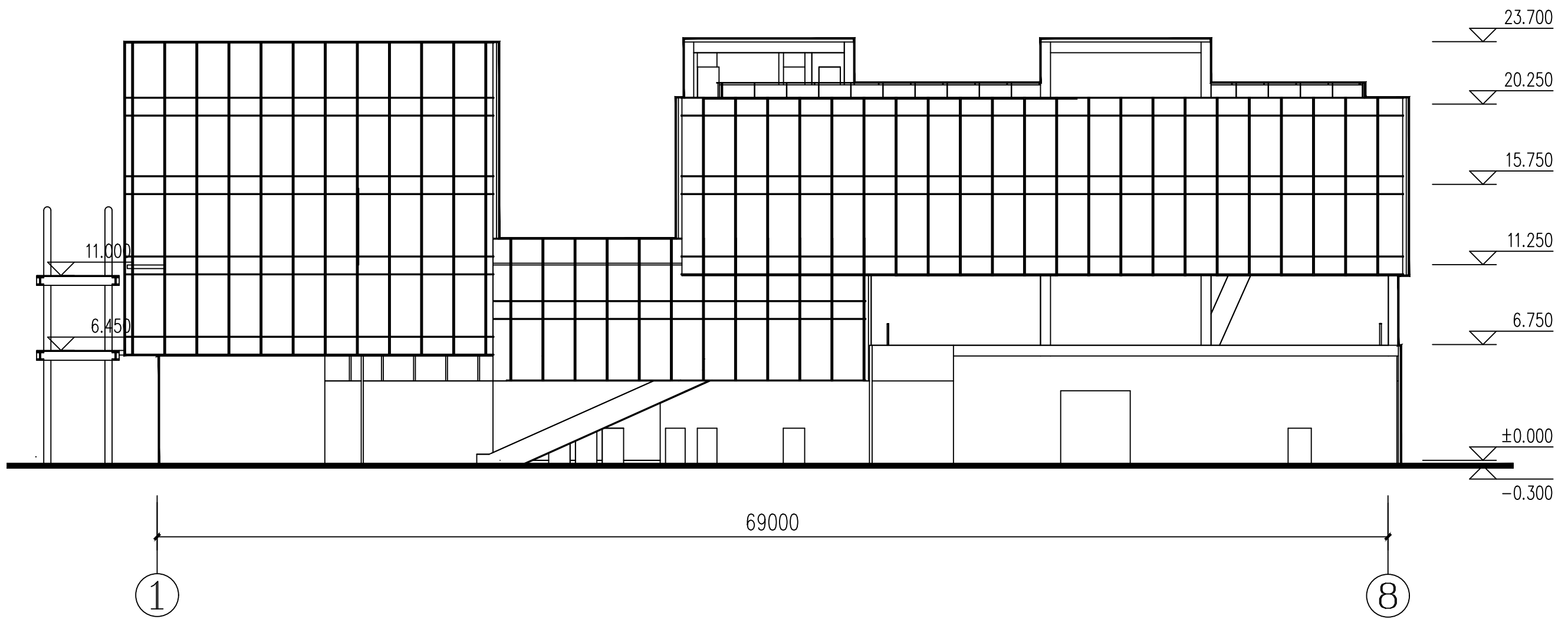
①—⑧立面图 1:250
