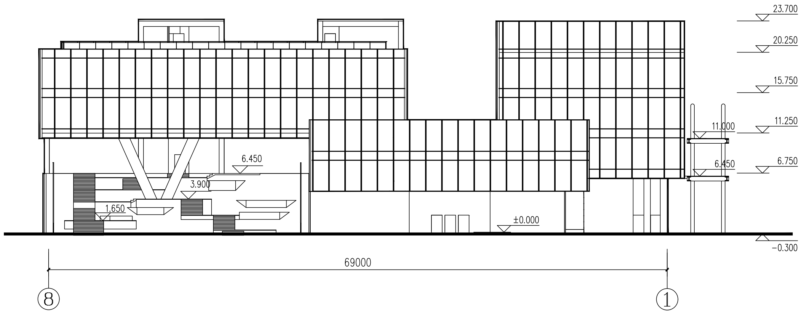
⑧—①立面图 1:250
