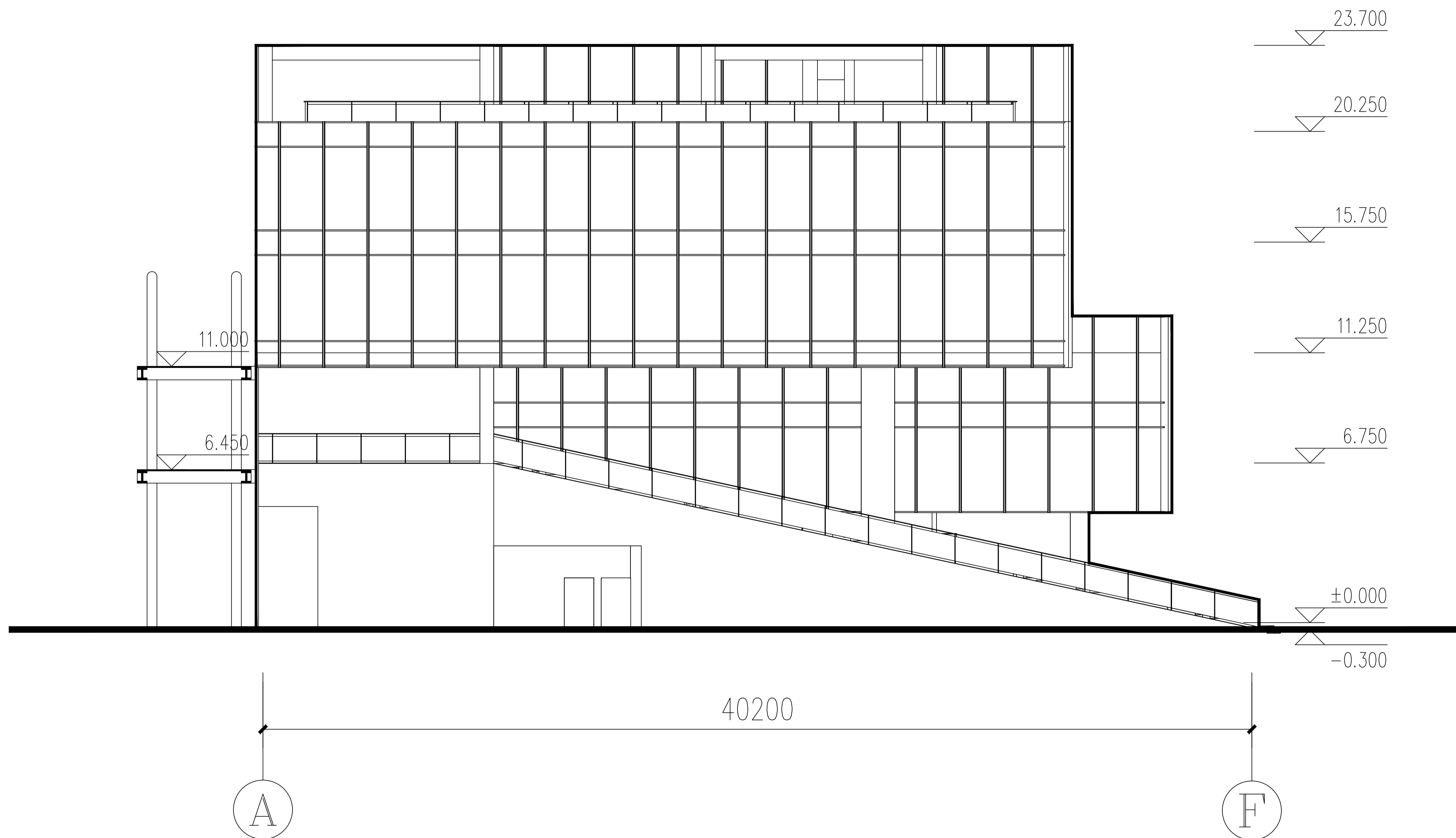
A—F 立面图 1:200
