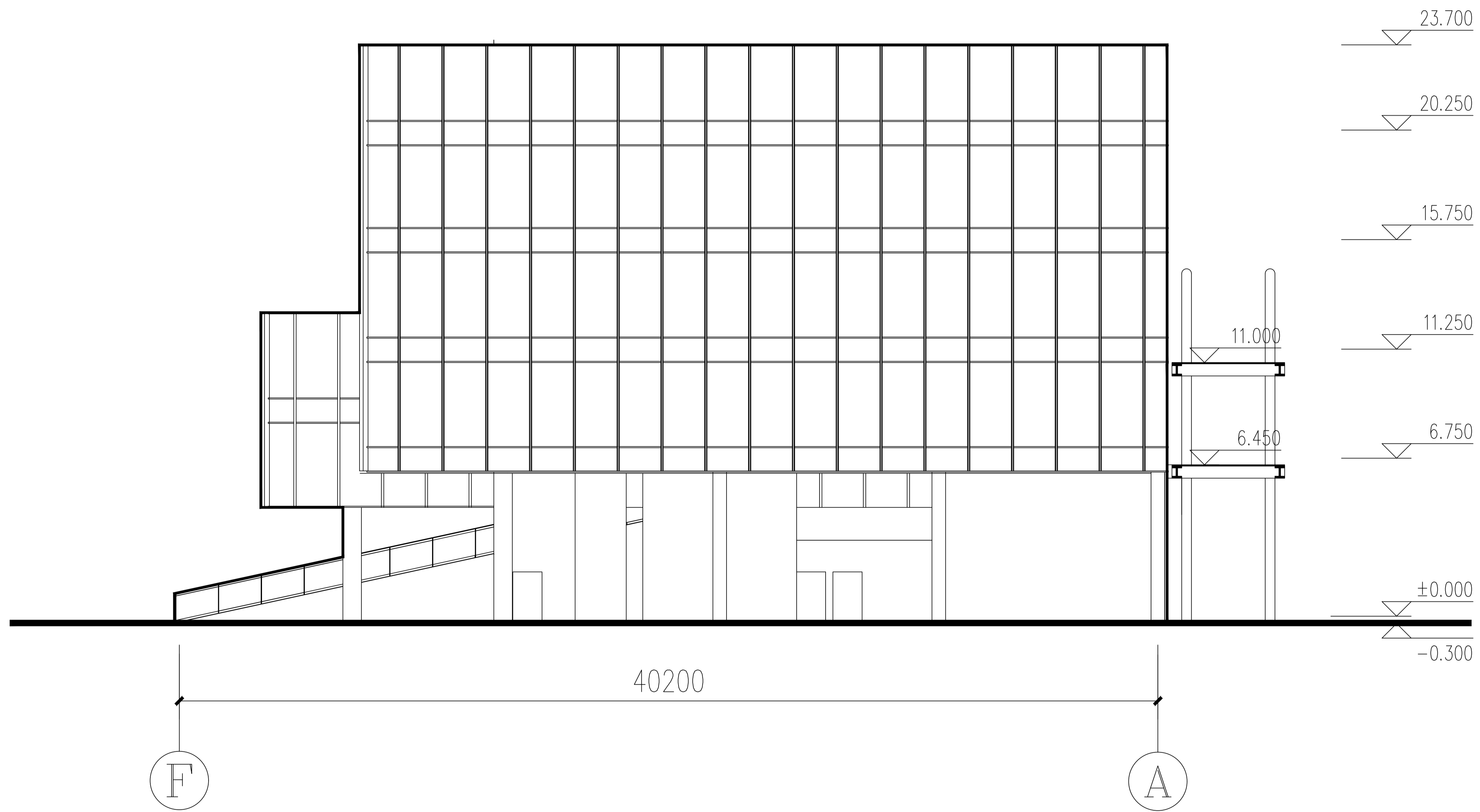
F—A 立面图 1:200
