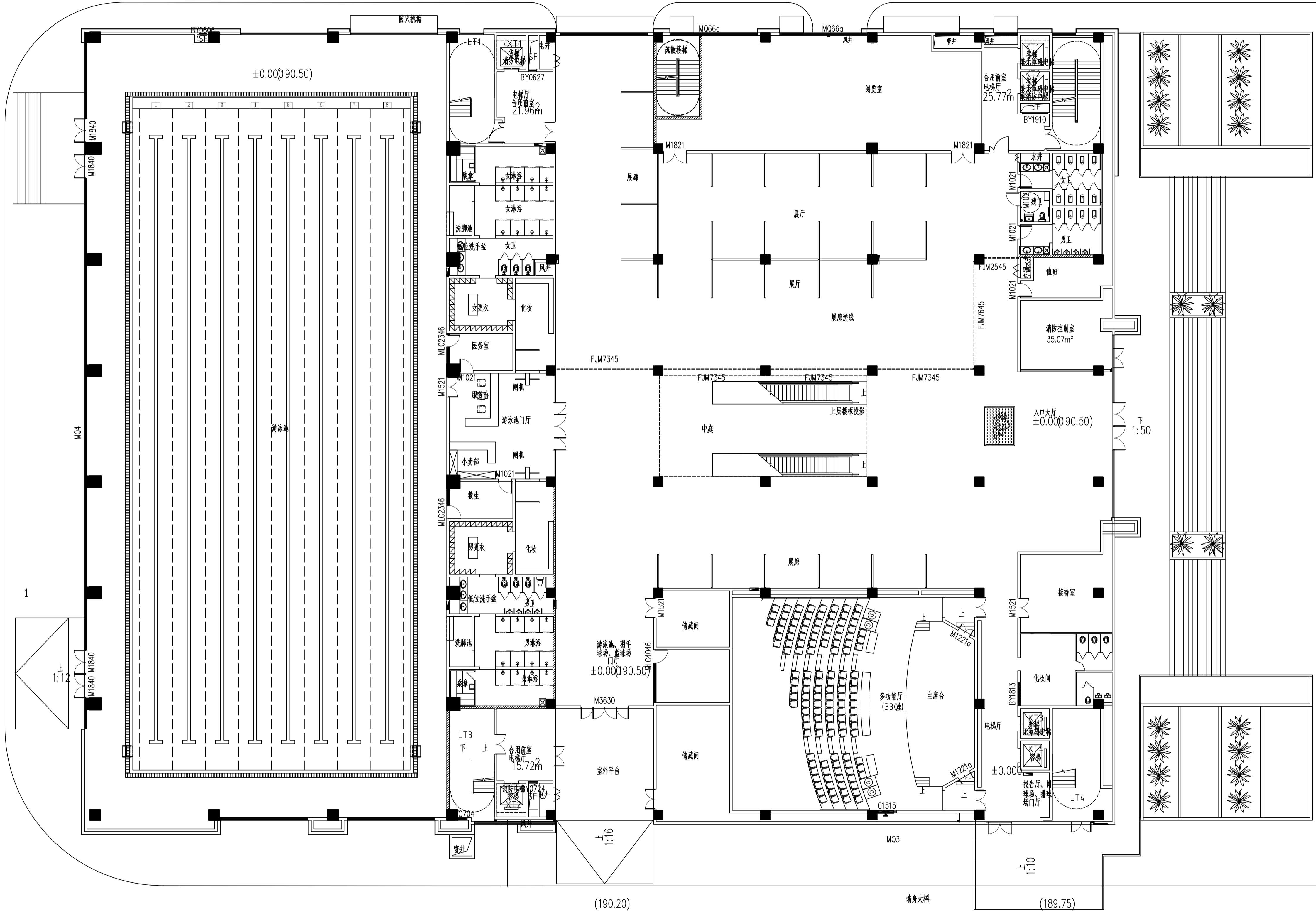
一层平面图
