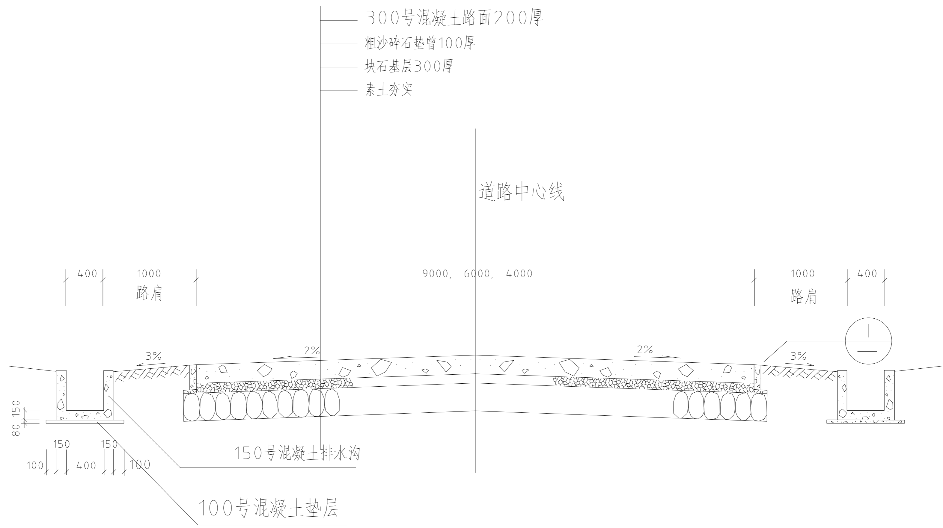
道路构造断面图
