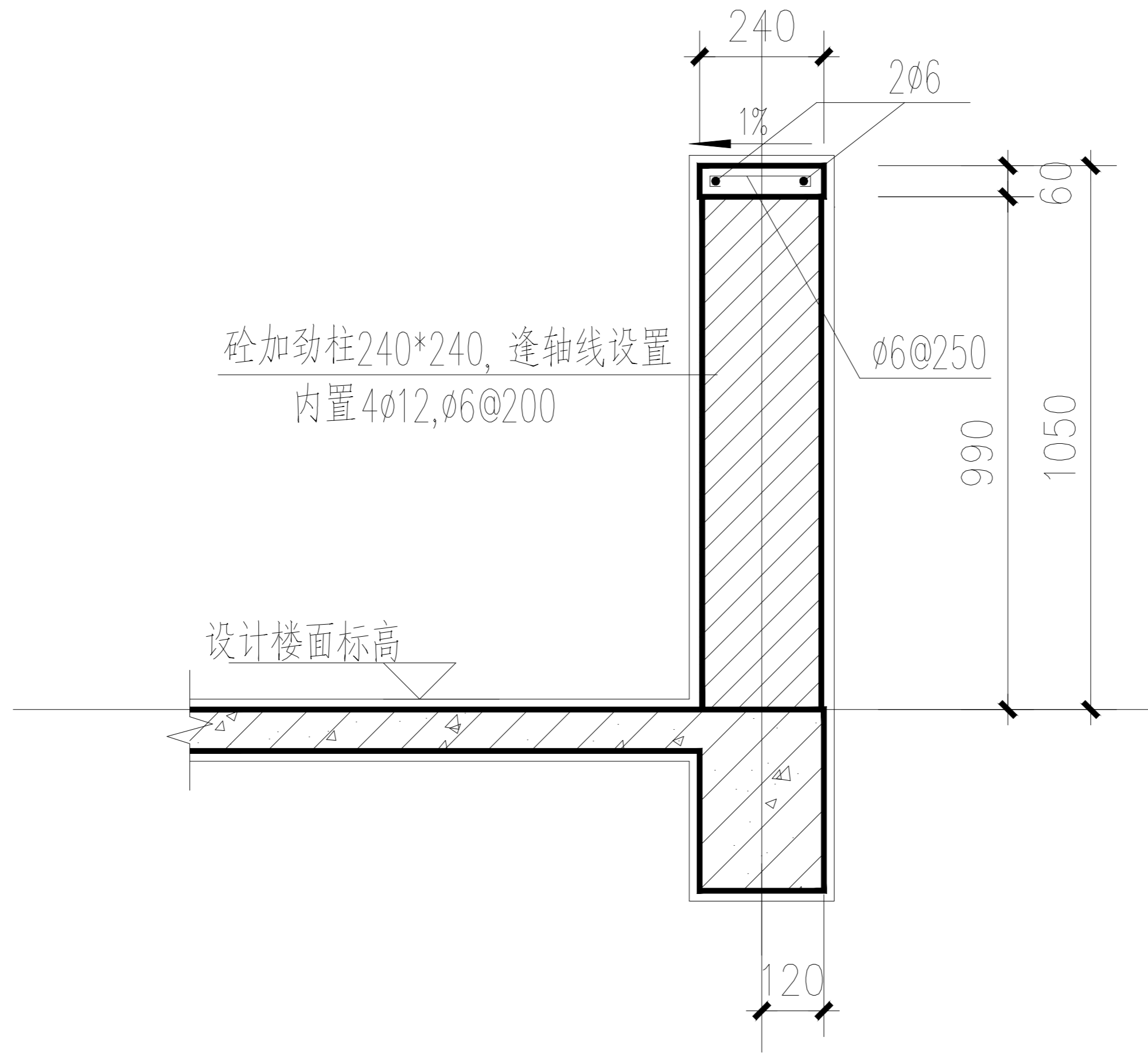
240厚砖砌栏板大样1:20
