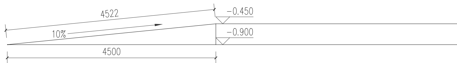
无障碍坡道示意图 1:20
