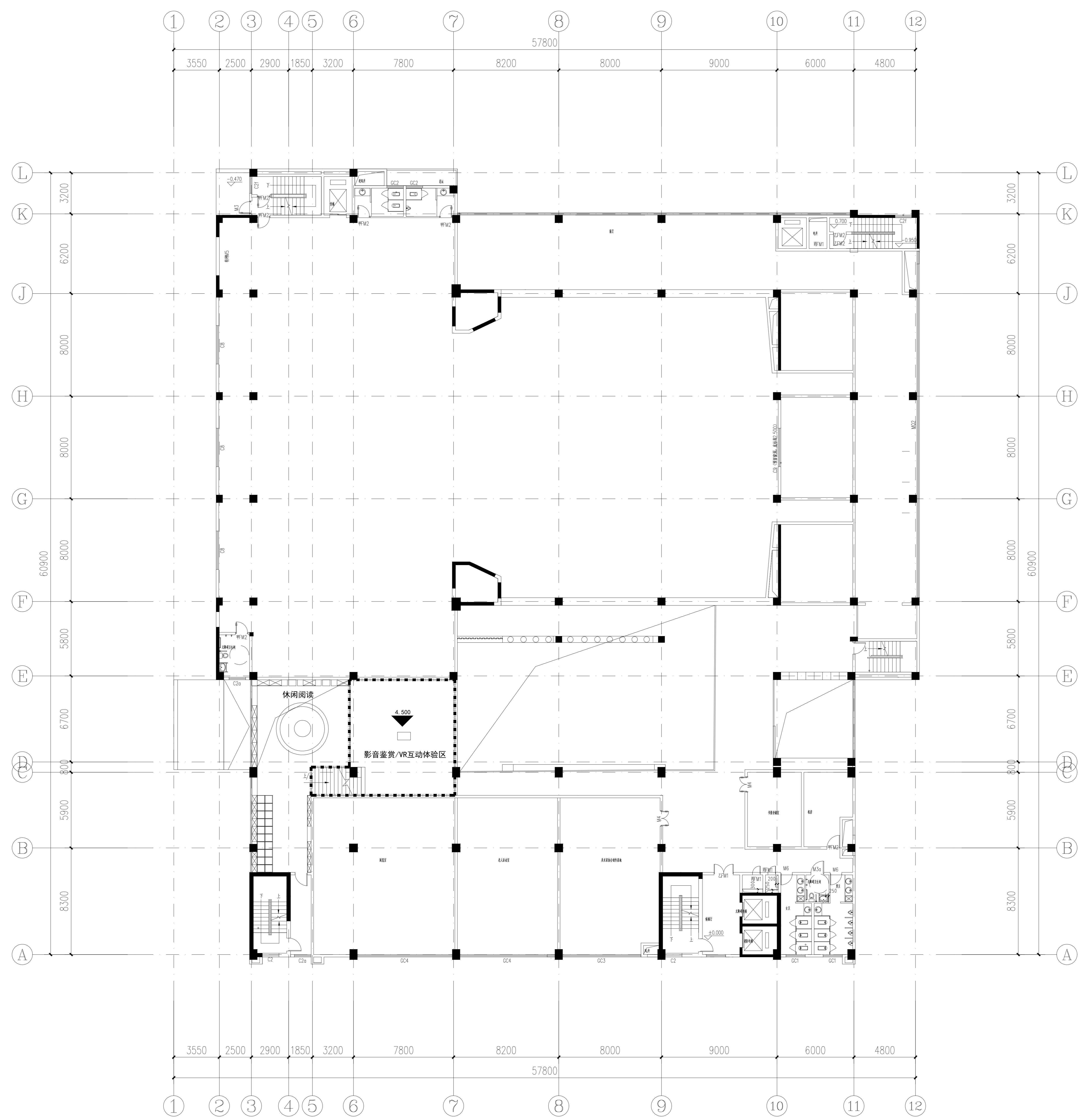
三层平面布置图1:100
