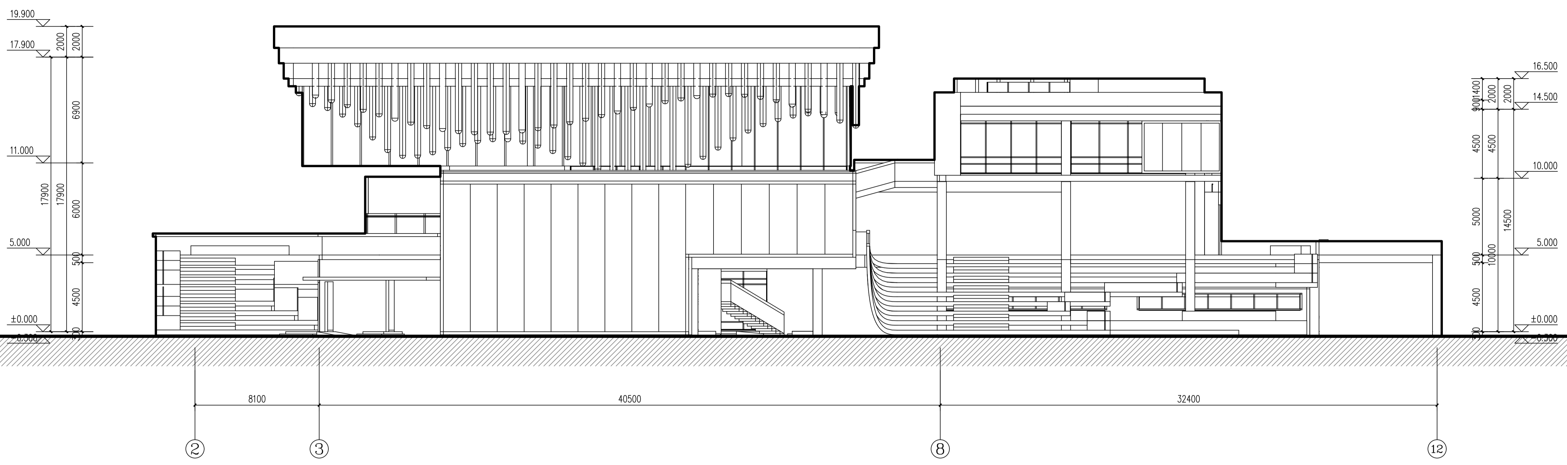
②-⑫轴立面图 1:150
