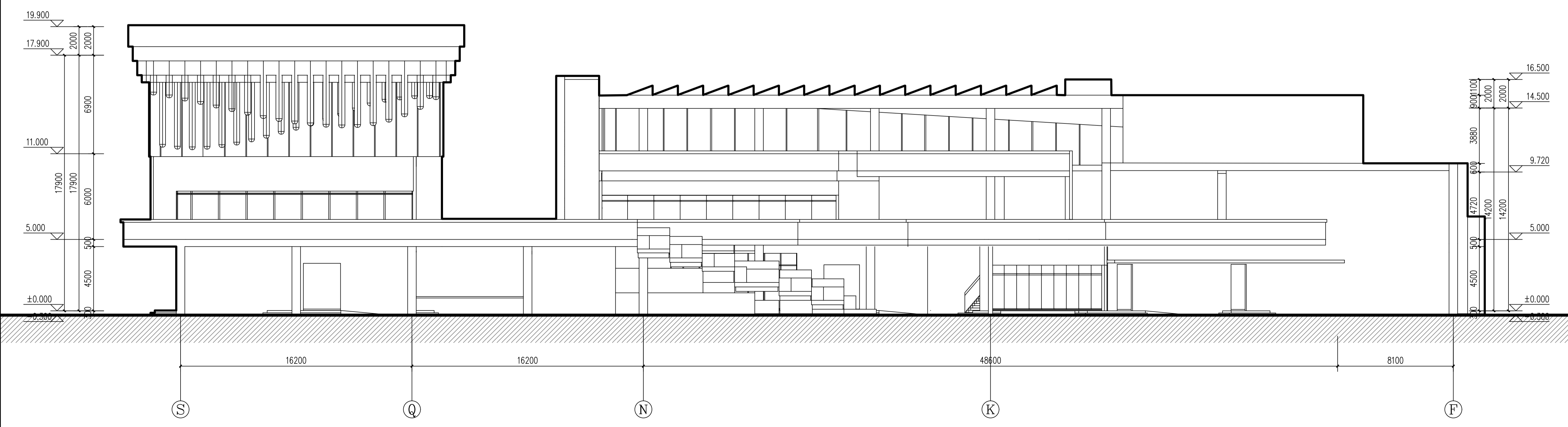
S-F轴立面图:150
