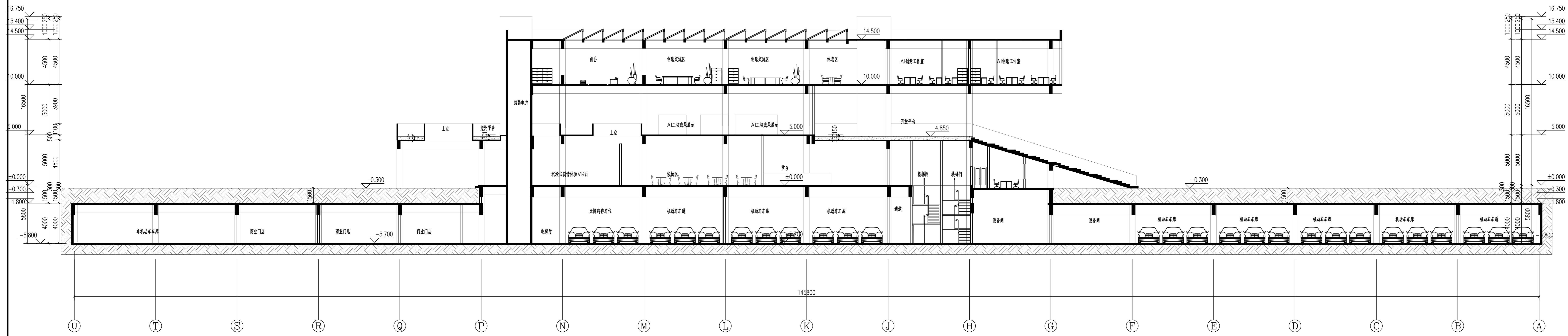
1-1剖面图 1:150
